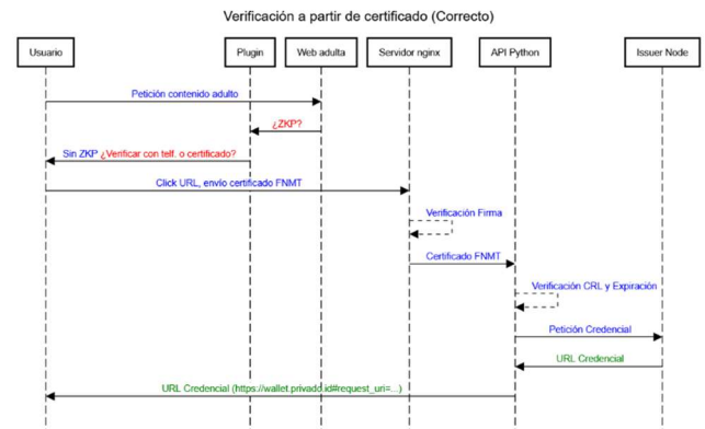
Fig. 4 Verificación a partir de certificado
