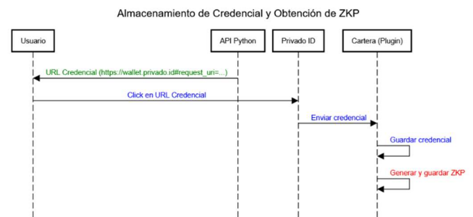
Fig. 5 Almacenamiento de credencial y Obtención de ZKP
