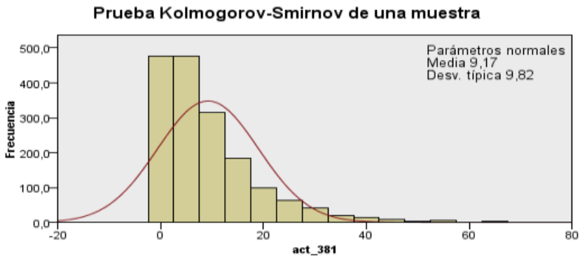
Gráf. 4.13 función de densidad de la actividad 381
