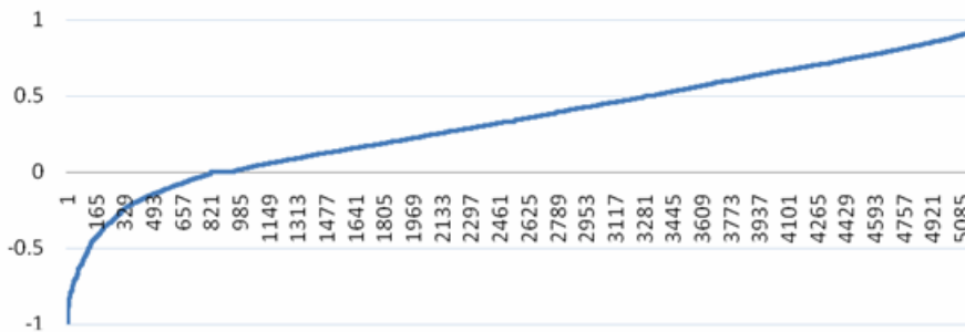
Gráf. 4.8 Valor de q^{(i)} para cada hogar
