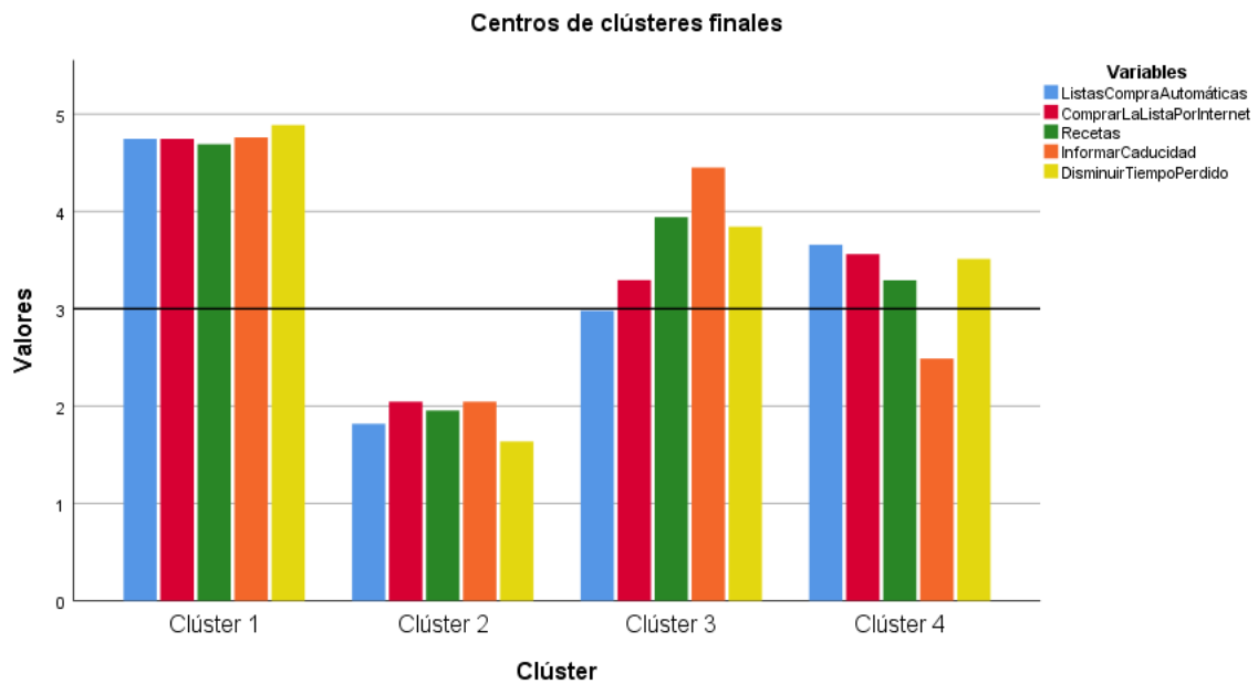
Gráfico 20- Representación gráfica de los centroides finales
