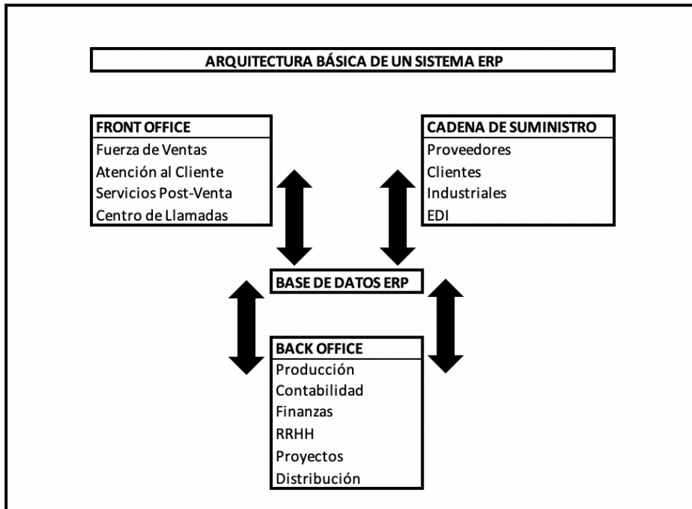
Figura 2: Arquitectura básica de un sistema ERP
