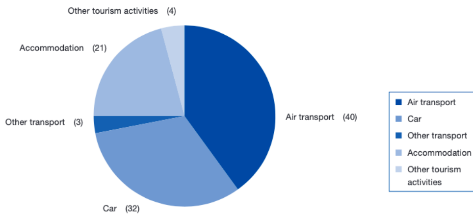
Figura 5. Contribución de varios subsectores a las emisiones de CO 2 del turismo, 2005 (%)
