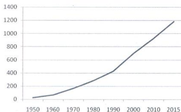
Figura 4. Evolución del número de turistas internacionales entre 1950 y 2015 (en millones)
