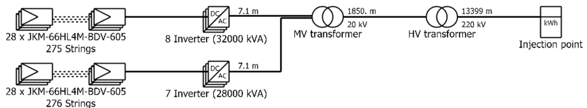
Figura 15. Unifilar resumen de la instalación
