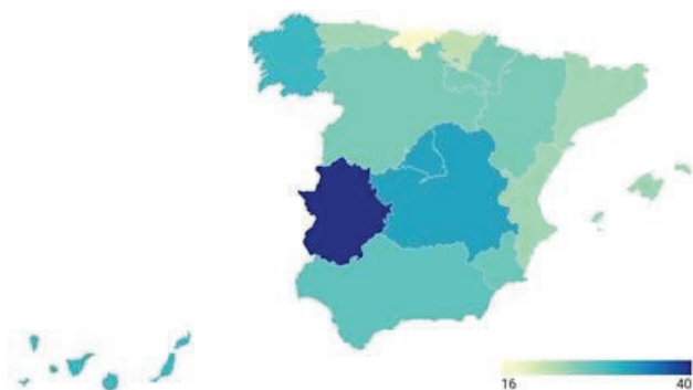
Figura AII.2. Participación de la energía eólica [%] en la hibridación eólica/fotovoltaica para alcanzar el LCOH mostrado en la Figura AII.1.
