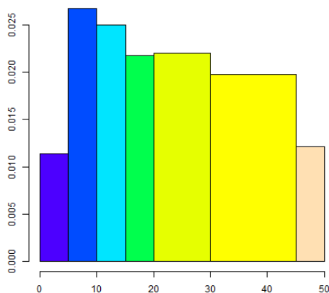
Figura 1.4: Histograma.
