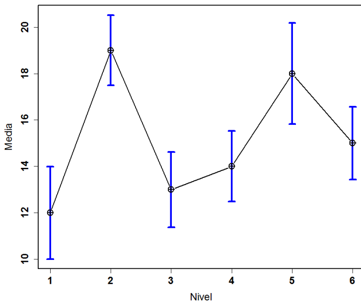
Figura 11.6: Intervalos de confianza (ajustados por Bonferroni) para las medias del Ejemplo 11.6.4.
