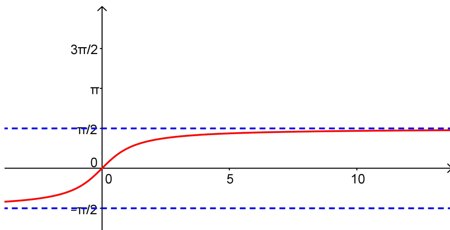
Figura 5.10: Gráfica de la función F(x) del Ejemplo 5.4.3.
