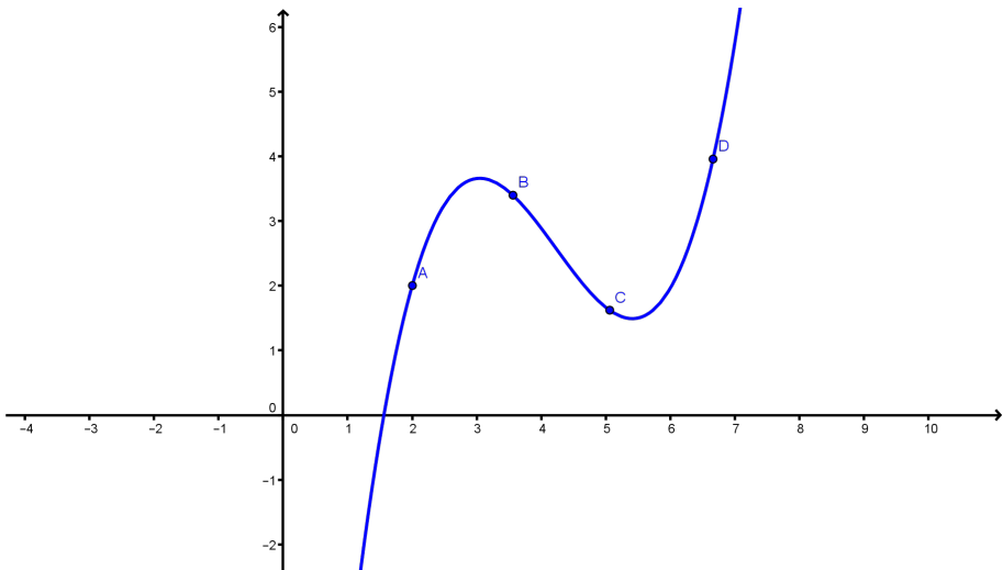
Figura 10.4: Interpolación.
