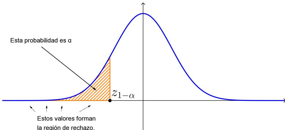
Figura 7.4: Región de rechazo para H_0 = \{\mu \geq \mu_0\} .
