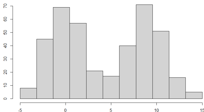
Figura 2.1: Un conjunto de datos bimodal.
