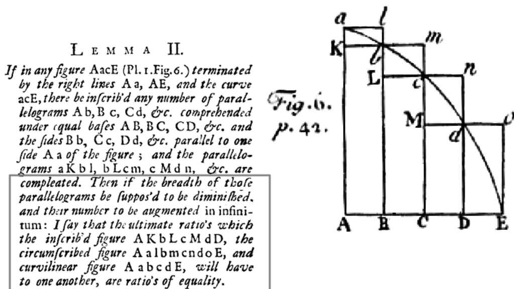
Figura 5.4: Un fragmento de los Principia Mathematica de Newton.
