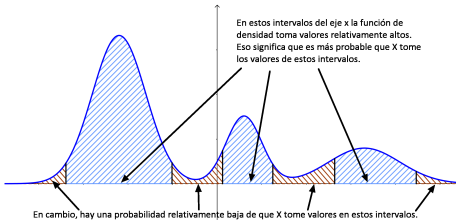
Figura 5.13: La altura de la función de densidad indica los valores de X con más probabilidad.
