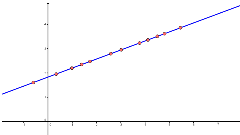
Figura 10.8: El único caso en el que EC = 0 es el de los puntos situados en una recta.
