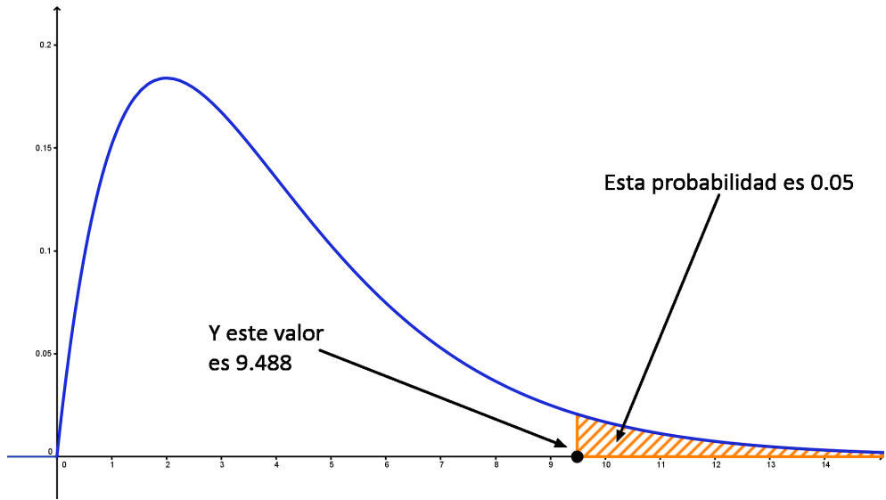
Figura 6.14: Problema inverso de probabilidad ( p_0 = 0.05 ) para \chi_4^2 , cola derecha.
