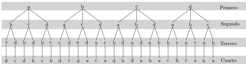
Figura 3.10: Posibles colas
