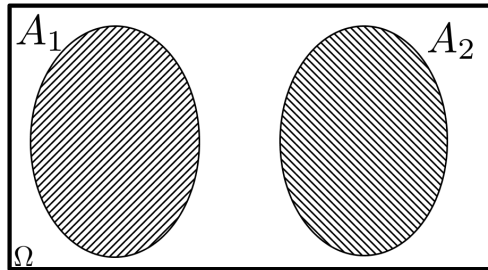
Figura 3.5: Diagrama para la intersección de dos sucesos
