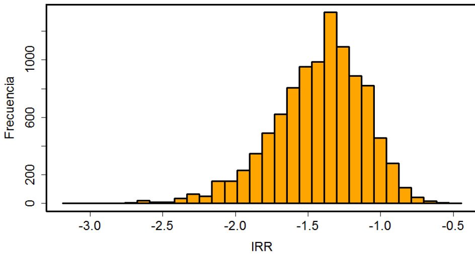
Figura 9.8: Simulación con 10000 muestras, de tamaño n = 50 , con p_1 = 0.2 y p_2 = 0.8 , en el Ejemplo 9.4.2. (a) Distribución muestral del riesgo relativo. (b) Distribución muestral del logaritmo del riesgo relativo.
