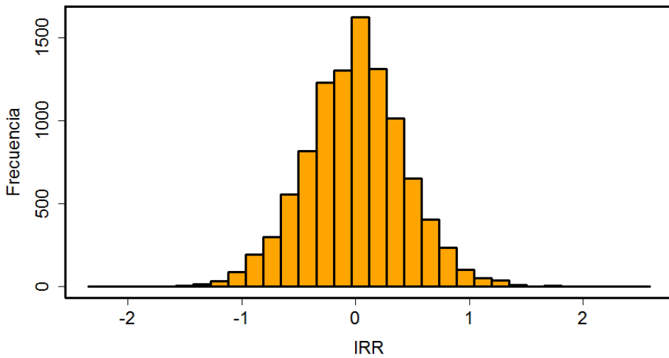
Figura 9.6: Simulación con 10000 muestras, de tamaño n = 50 , con p_1 = p_2 = 0.2 , en el Ejemplo 9.4.2. (a) Distribución muestral del riesgo relativo. (b) Distribución muestral del logaritmo del riesgo relativo.
