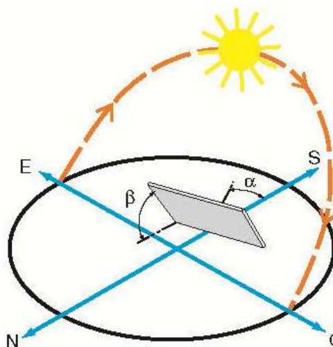
Figura 74. Parámetros de diseño PV: pendientes y azimut.
