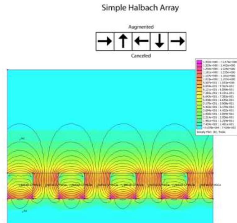
Figura 24. a) Esquema Matriz Halbach [42]. b) Líneas de campo magnético. Fuente: Gaia Final Design.
