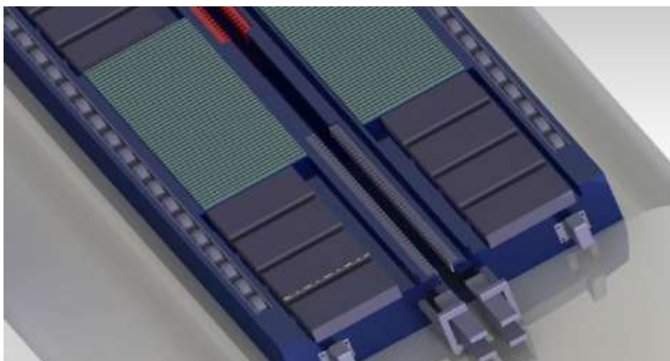
Figura 20. Vista en detalle del sistema de estabilización activo. Fuente: Gaia Final Design.
