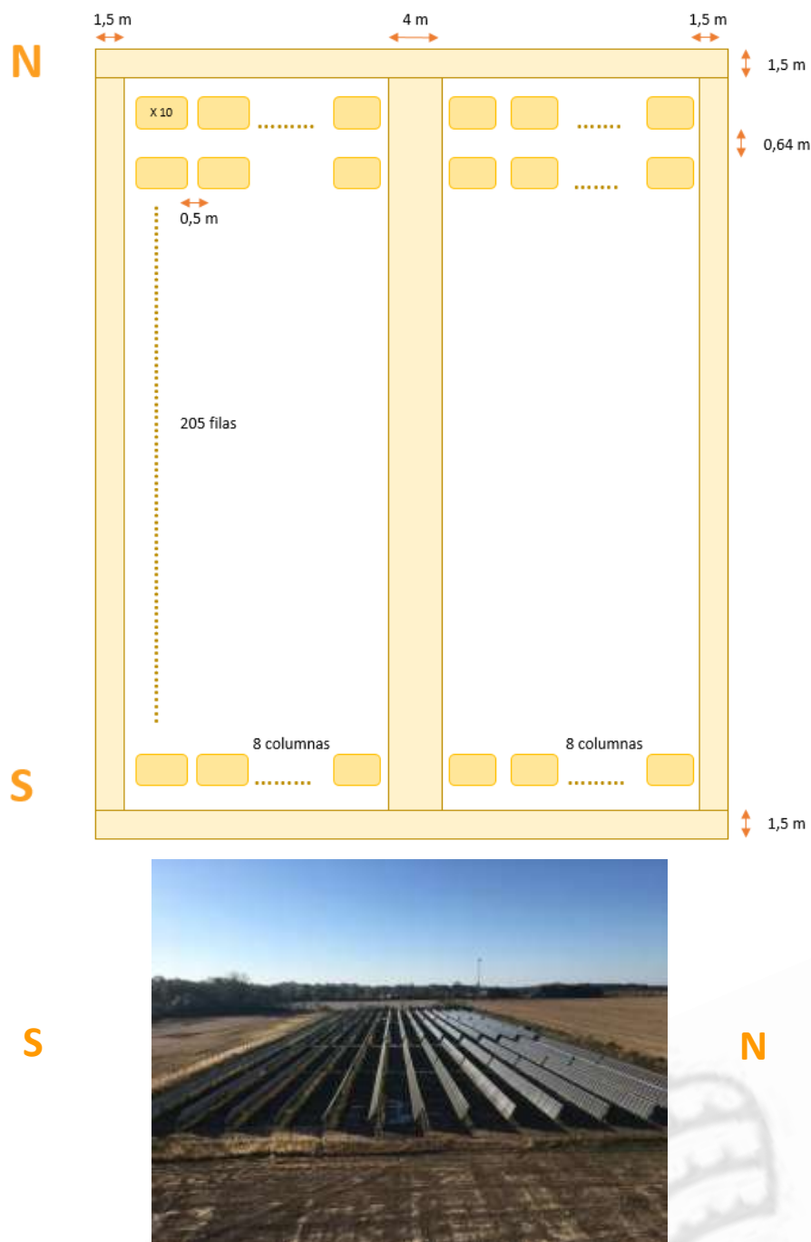
Figura 79 Distribución de los paneles fotovoltaicos en el sola. Vista en planta y estimación de la vista en perfil. Fuente: Elaboración propia.
