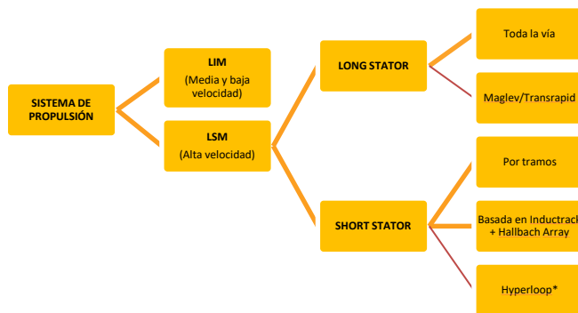
Figura 7. Resumen sistema de propulsión. Fuente: Elaboración propia.
