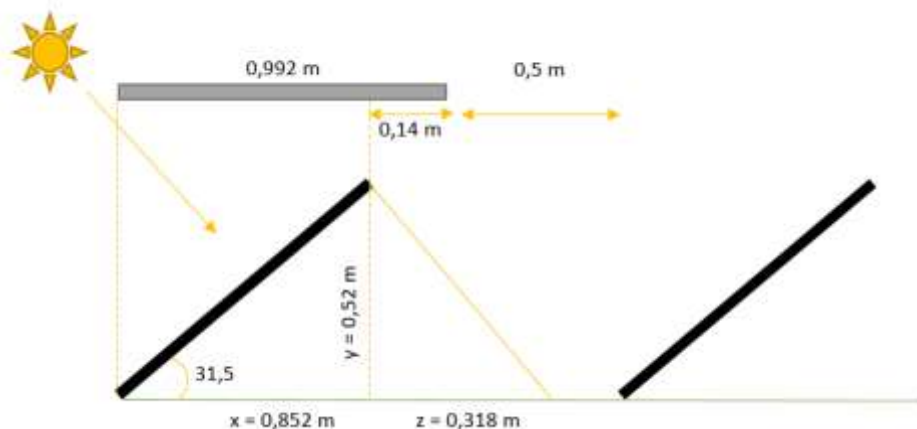
Figura 80. Vista en perfil disposición de las placas solares. Fuente: Elaboración propia.
