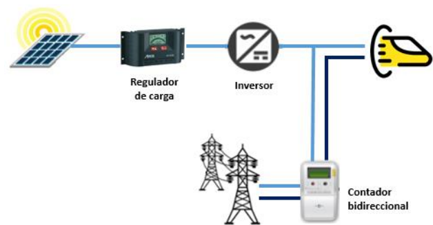
Figura 11. Esquema de la instalación modo autoconsumo. Fuente: Elaboración propia.
