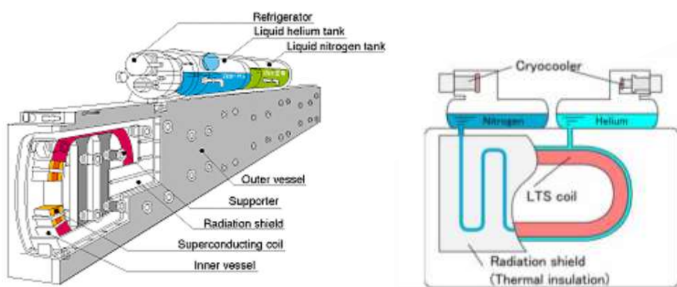
Figura 31. Esquema sistema de refrigeración superconductores Maglev. Fuente: [59]
