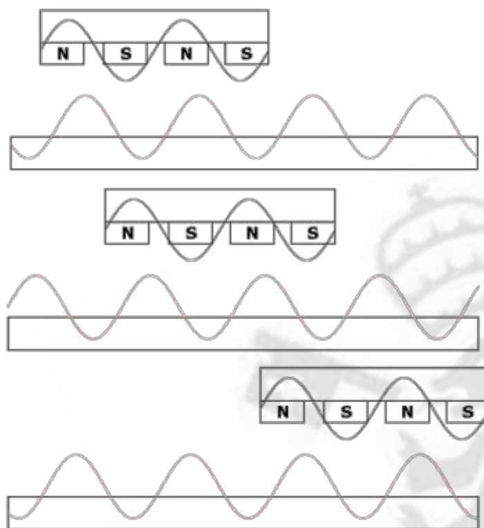
Figura 22. Esquema funcionamiento sistema de propulsión LSM. Fuente: Coasters and more.
