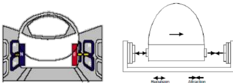
Figura 19. Esquema de las vías laterales basadas en electroimanes. Fuente: [10]
