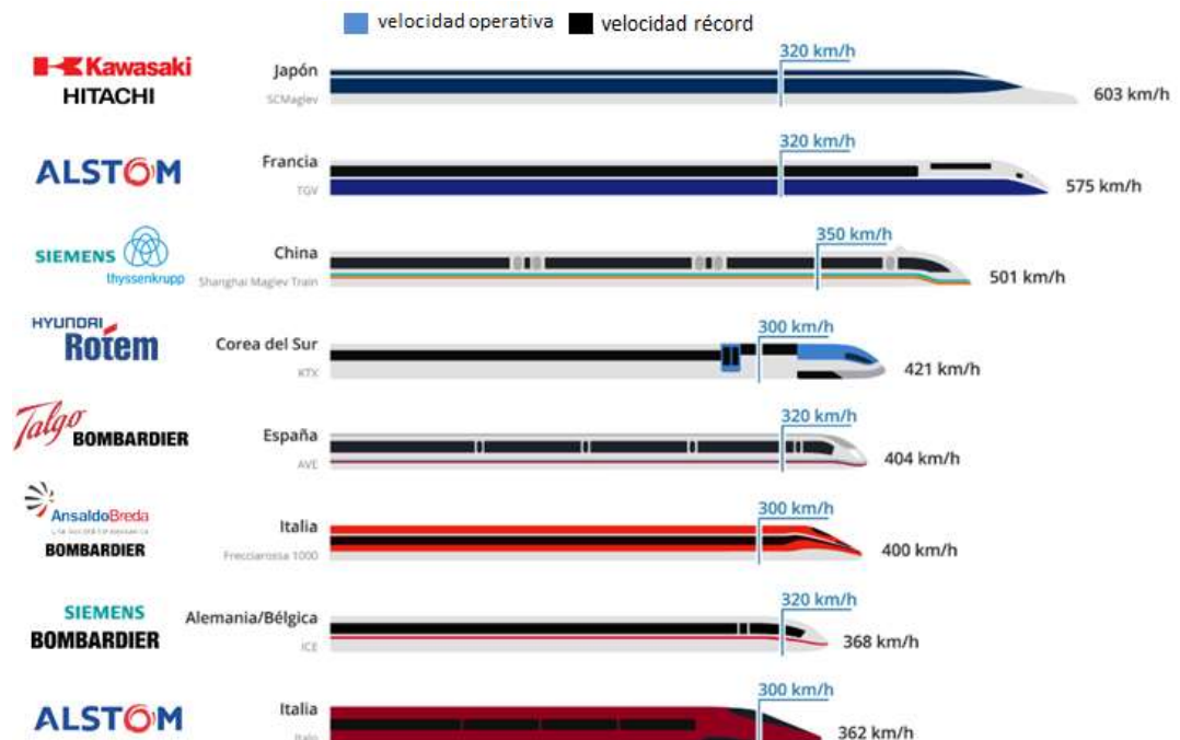
Figura 10. Comparativa trenes de alta velocidad. Fuente: GoEuro. [28].
