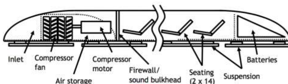
Figura 14. Esquema de la cápsula de pasajeros. Fuente: Hyperloop Alpha. [25]
