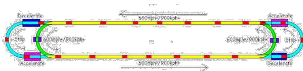
Figura 28. Esquema propuesto para el sistema de aceleración y deceleración de Hyperloop. [2]
