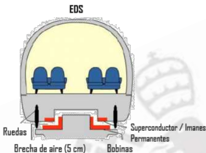
Figura 17. Esquema de suspensión electrodinámica, EDS.
