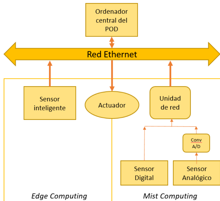
Figura 30. Arquitectura de la comunicación interna. Fuente: Elaboración propia.
