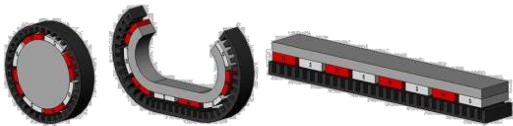
Figura 21. Esquema constructivo de la evolución del motor de inducción convencional al lineal. Fuente: Motion Control [58].
