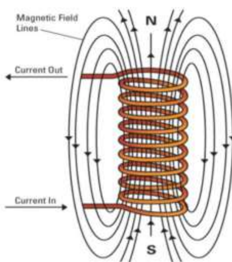
Figura 15. Funcionamiento de un electroimán. Fuente: [18].
