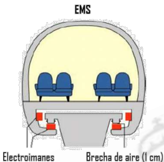
Figura 16. Esquema de suspensión electromagnética, EMS.
