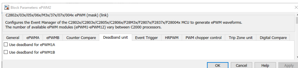
Figura 6.43: Configuración pestaña Deadband Unit para obtención de señales por PWM.
