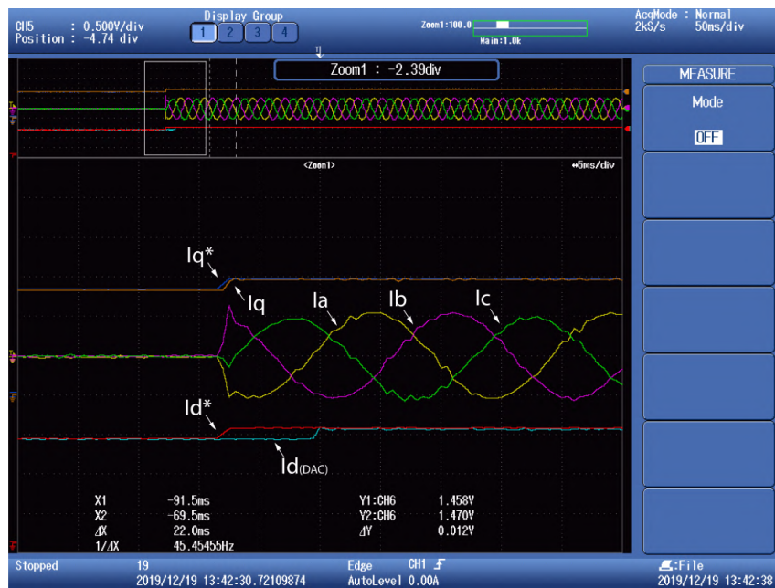
Figura 8: Corrientes trifásicas por las bobinas. Respuesta temporal de corriente de eje d y eje q. Aplicación de las referencias de manera simultanea. La identificación de las señales se muestran en detalle en la figura.
