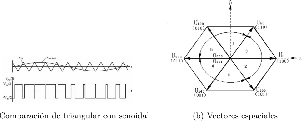
Figura 2: Obtención de señales PWM
