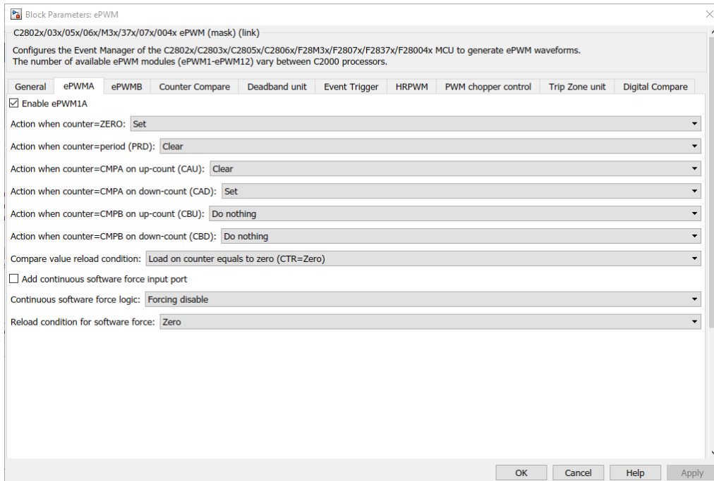
Figura 6.33: Configuración ePWMxA.
