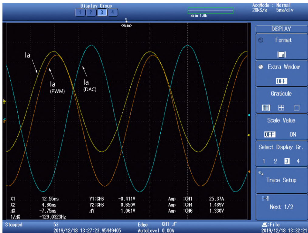
Figura 6.49: Corriente por una fase, salida por el DAC, por el PWM y medida con pinza amperimétrica.
