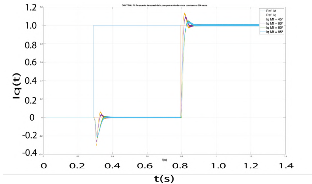
Figura 5.18: Respuesta temporal de I_q con pulsación de cruce constante con el control PI en tiempo continuo. Pulso de I_d = 1 en 0.3s. Pulso de I_q = 1 en 0.8s.
