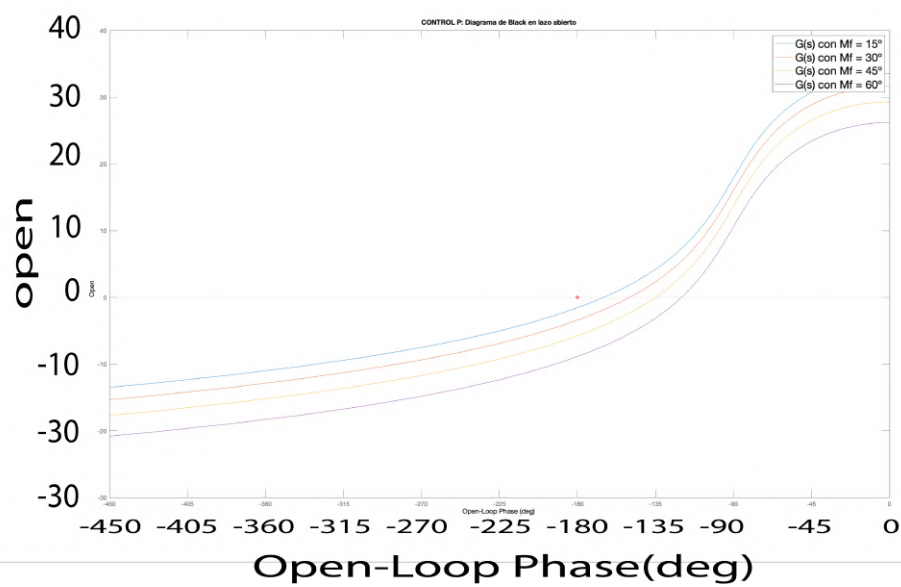
Figura 5.11: Respuesta en frecuencia de lazo abierto de un Control P en tiempo continuo.
