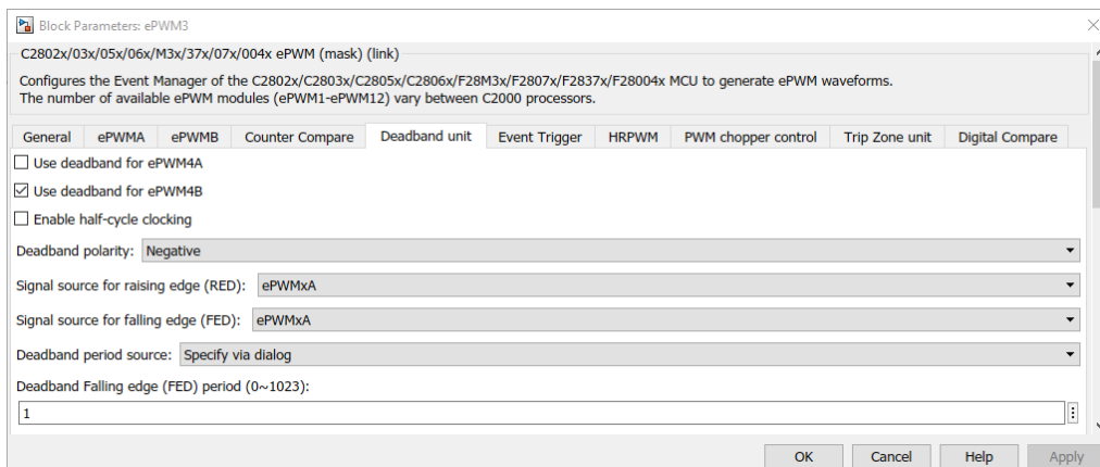
Figura 6.37: Configuración ePWMxB desde el DeadBand Unit .
