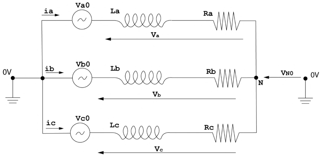
Figura 4.1: Esquema vectorial del circuito. V_{a0} , V_{b0} y V_{c0} son las tensiones de salida del inversor. V_a , V_b y V_c las tensiones que determina el control e i_a , i_b e i_c las variables medidas.
