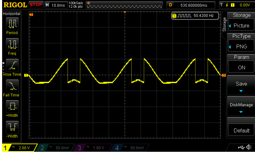
Figura 6.51: Señal saturada por la salida del DAC.
