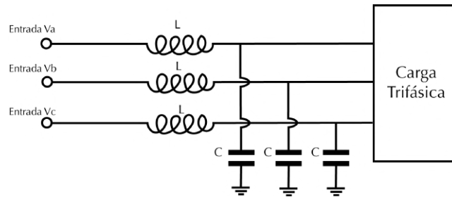
Figura 3.9: Filtro en LC.
