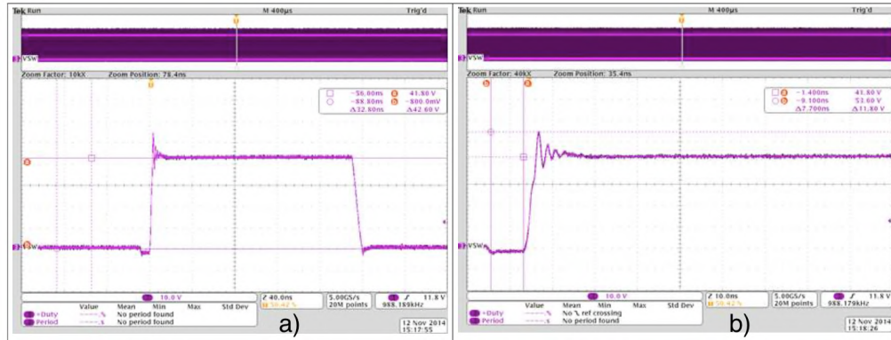
Figura 6.16: a) apagado y b) encendido del LMG5200 [49].
