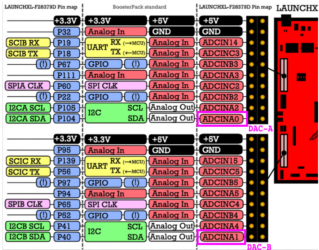
Figura 6.9: Vista de detalle de la tarjeta LAUNCHXL - F28379D Pinout lado izquierdo [45]. Se recuadran las salidas del DAC para las que existe un bloque en el toolbox de Simulink.
