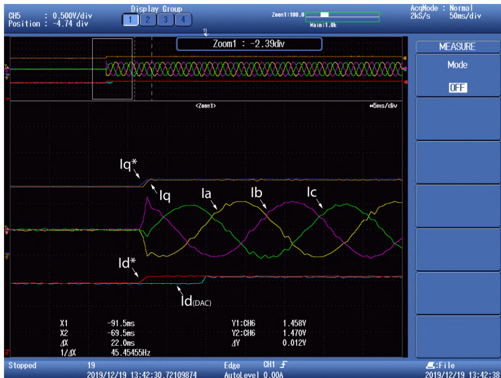
Figura 7.7: Corrientes trifásicas por las bobinas. Respuesta temporal de corriente de eje d y eje q. Aplicación de las referencias de manera simultánea. La identificación de las señales se muestran en detalle en la figura.
