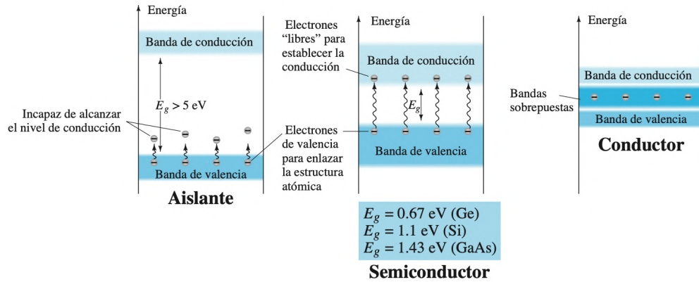
Figura 2.8: Banda de conducción de materiales semiconductores[13].
