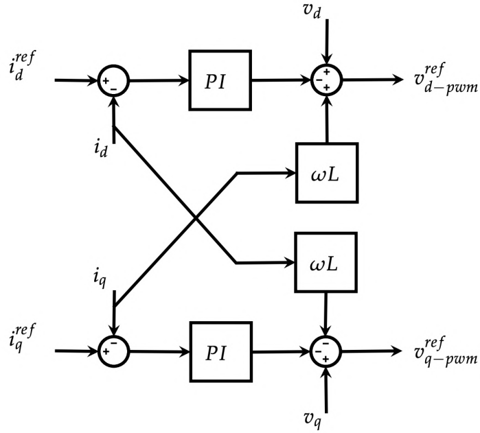
Figura 4.4: Diagrama de control de corriente en ejes d-q [25]
