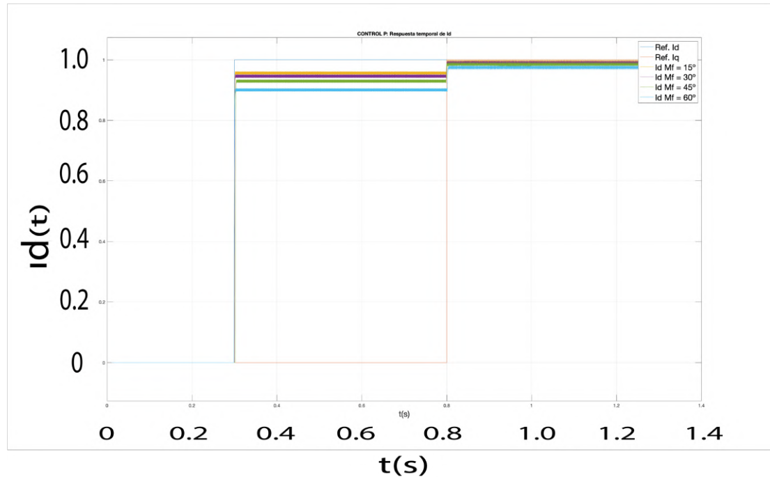
Figura 5.9: Respuesta temporal de eje d de un Control P en tiempo continuo. Pulso de I_d = 1 en 0.3s. Pulso de I_q = 1 en 0.8s.
