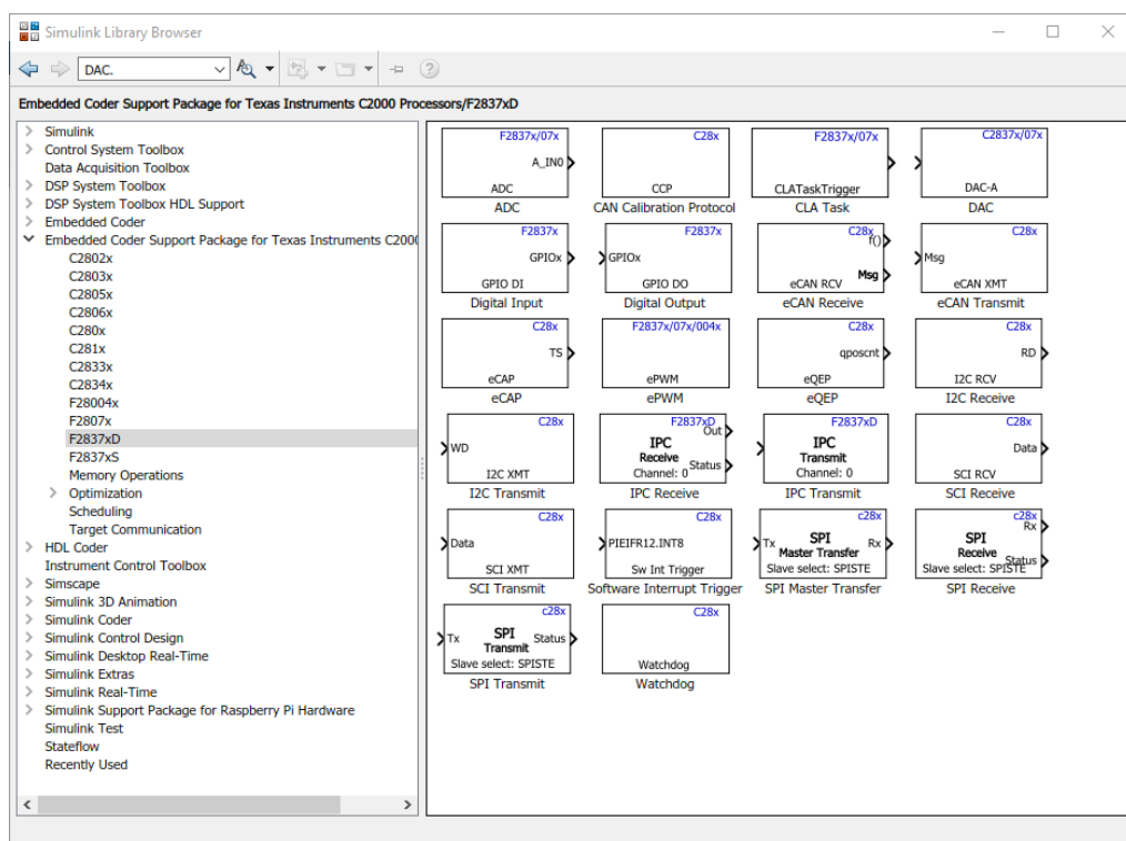
Figura 6.12: Toolbox para el LaunchPad F2837xD de Texas Instruments.[46]
