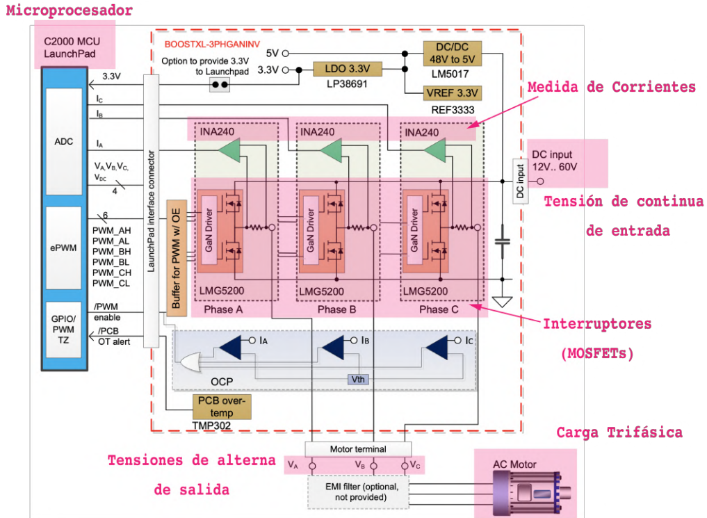
Figura 2.15: Diagrama funcional del VSC utilizado en el prototipo.
