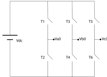
Figura 1: Esquema de un inversor trifásico. V_{dc} es la tensión continua de entrada, V_{a0} , V_{b0} y V_{c0} son las tensiones alternas de salida.
