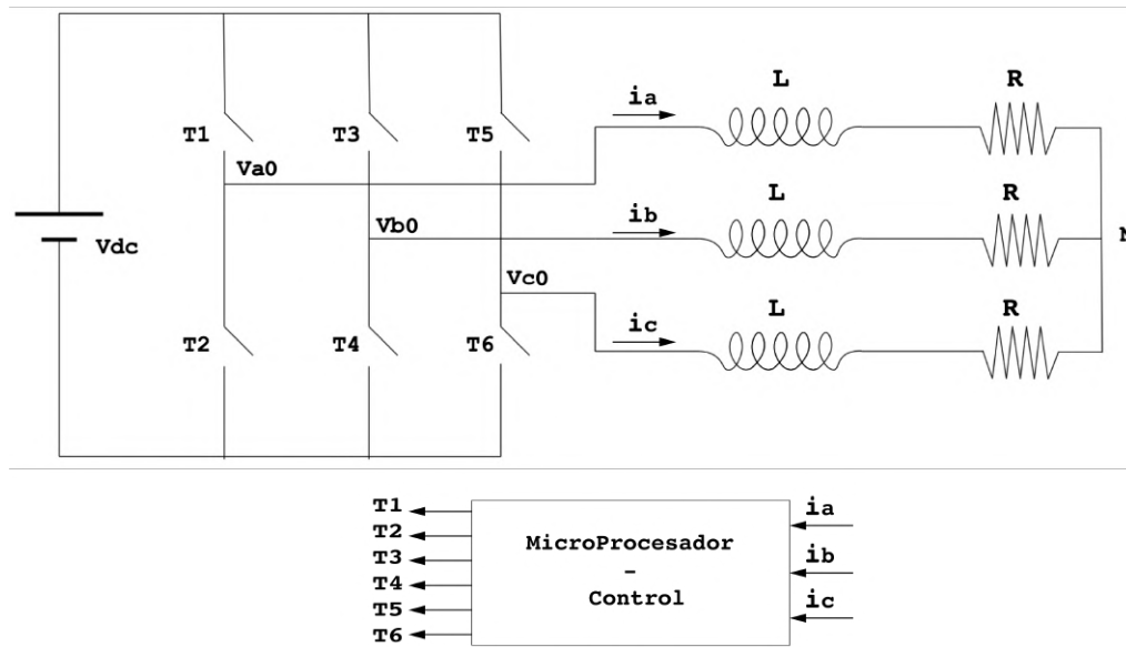
Figura 2.14: Esquema de un VSC alimentando una carga. V_{dc} es la tensión de continua de entrada gobernable. T1 a T6 son los interruptores disparados con el microprocesador. V_{a0} , V_{b0} y V_{c0} son las tensiones alternas de salida e i_a , i_b e i_c las corrientes por la carga. L y R es la carga que se alimenta.
