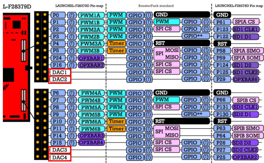
Figura 6.10: Vista de detalle de la tarjeta LAUNCHXL - F28379D Pinout lado derecho [45]. Se recuadran los pines para los que no existe un bloque específico de Simulink y no pueden utilizarse con dicha librería como DAC.
