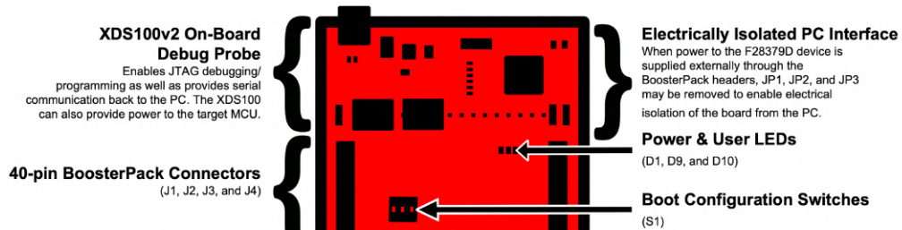
Figura 6.7: Vista en detalle parte superior tarjeta LAUNCHXL - F28379D [44]
