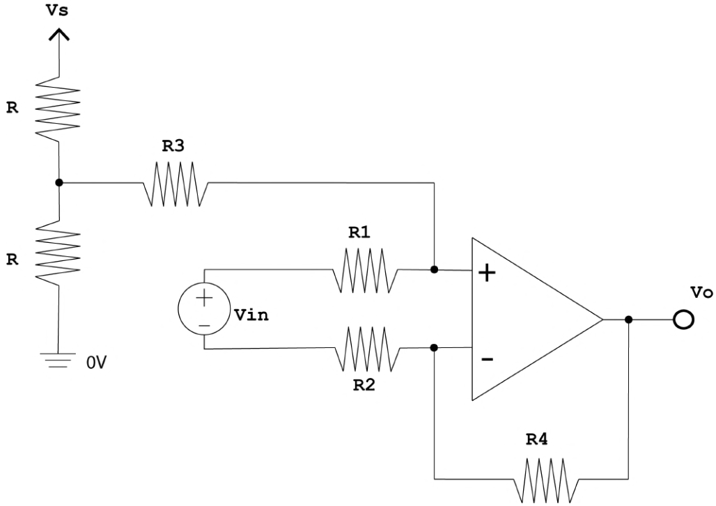
Figura 6.19: Circuito electrónico del INA240. [48]
