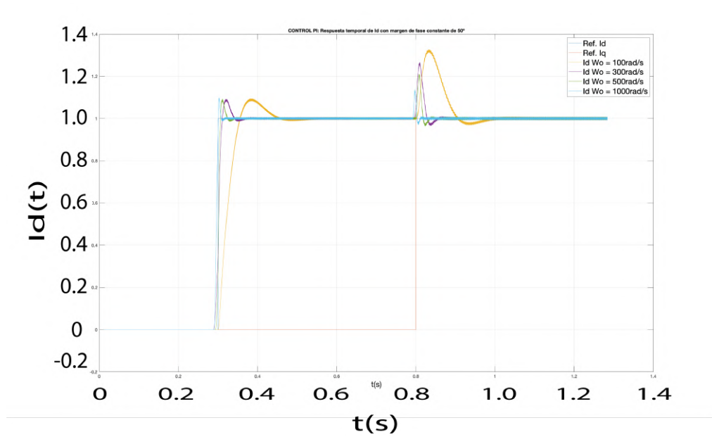
Figura 5.15: Respuesta temporal de I_d con margen de fase constante con el control PI en tiempo continuo. Pulso de I_d = 1 en 0.3s. Pulso de I_q = 1 en 0.8s.
