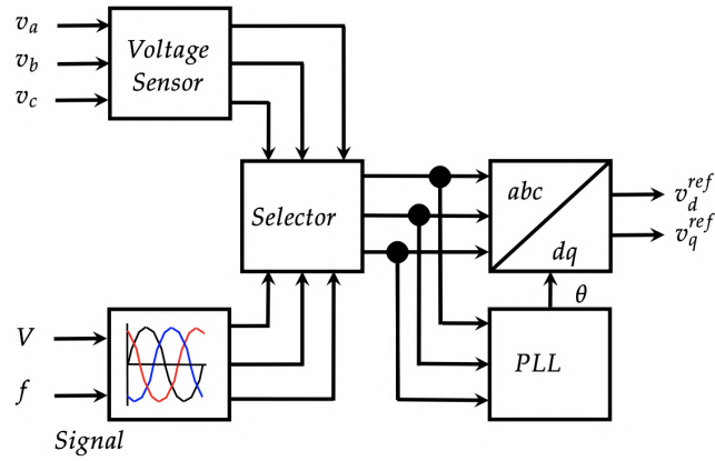
Figura 3.6: Modelo linealizado de un PLL [25].
