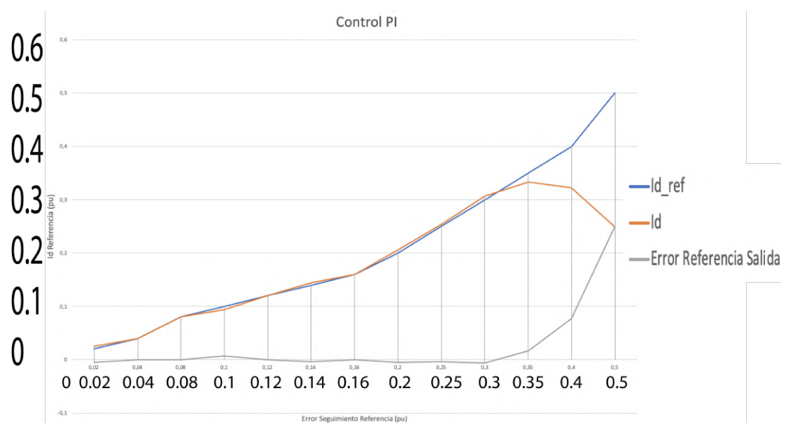
Figura 5.23: Gráfica de error de seguimiento de referencia de corriente de eje d con un Control PI. Implantación hardware. Los valores de los ejes están escalados a un 0.1 del valor real en pu. Se observa que la bobina satura para valores superiores a 3pu (Aprox. 6.1A).
