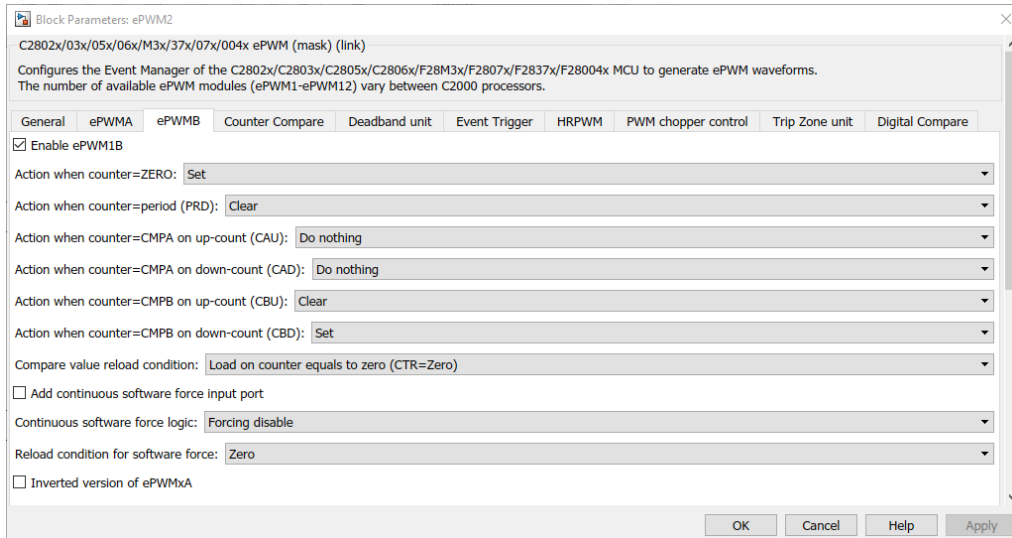
Figura 6.40: Configuración pestaña ePWMB para obtención de señales por PWM.
