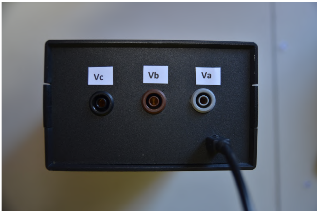
Figura 6.27: Encapsulado del VSC y Launchpad. Salidas de tensión alterna y conexión USB.
