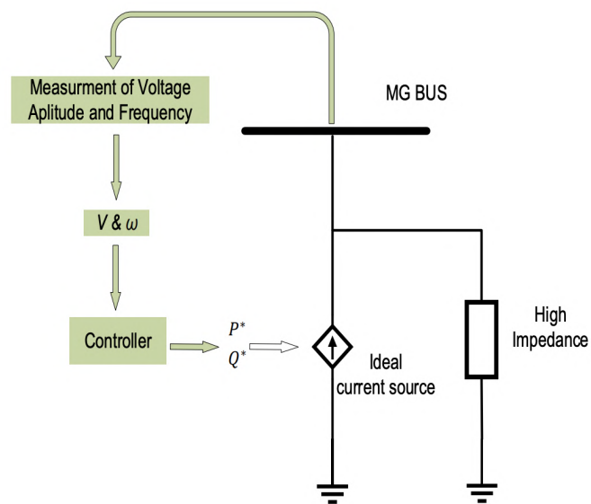
Figura 3.4: Diagrama de un convertidor en formato grid-supporting-feeding con modelo de fuente de corriente [23].
