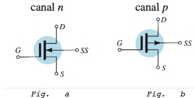
Figura 2.4: Diagrama de un transistor MOSFET a) canal n y b) canal p. [13]
