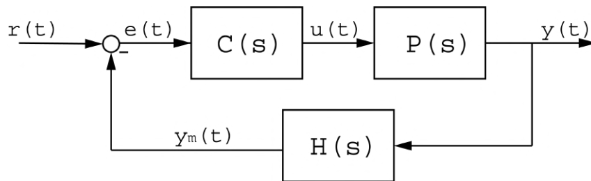
Figura 5.1: Diagrama de bloques de un control.
