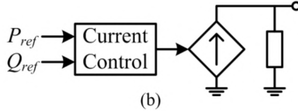
Figura 3.2: Diagrama de un convertidor en formato grid-feeding [22].
