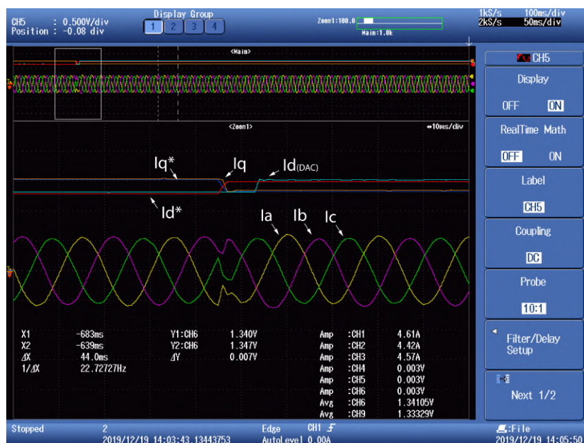
Figura 7.8: Corrientes trifásicas por las bobinas. Respuesta temporal de corriente de eje d y eje q inversamente aplicado. La identificación de las señales se muestran en detalle en la figura.
