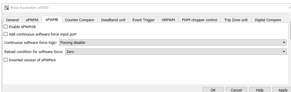
Figura 6.36: Configuración ePWMxB.
