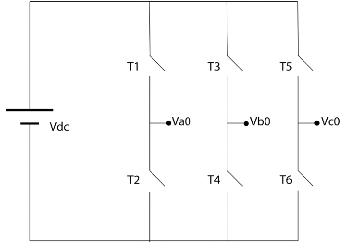
Figura 2.1: Esquema de un VSC trifásico. V_{dc} es la tensión continua de entrada, V_{a0} , V_{b0} y V_{c0} son las tensiones alternas de salida.
