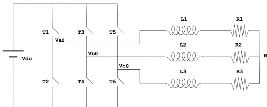
Figura 3.11: Esquema de inversor trifásico con carga RL.
