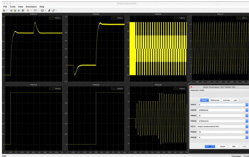
Figura 5.22: Scope de un simulador con un control PI. El bloque PID se implanta en tiempo discreto. Se puede observar en los saltos que se producen en los ejes dq cuando su referencia es nula, que las variaciones en eje q son perturbaciones en eje d y viceversa. Los valores del control de la simulación se recogen en la Tabla 5.4
