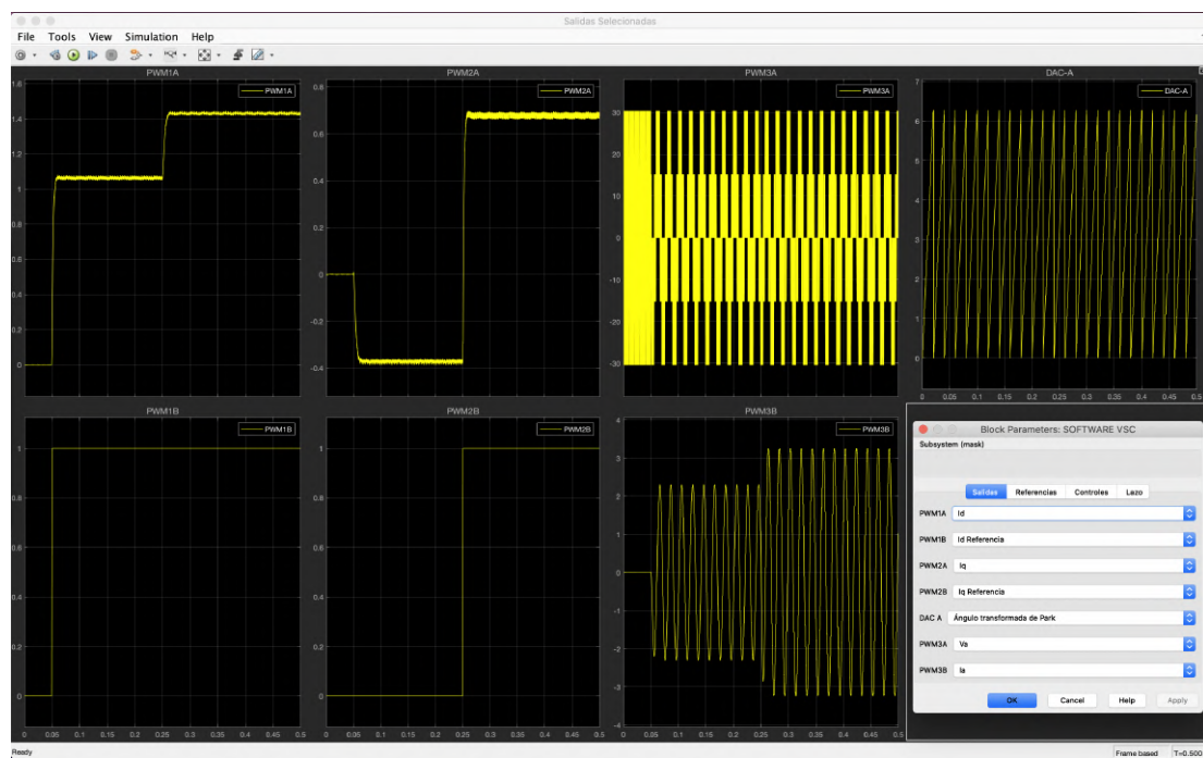
Figura 5.13: Scope de un simulador con un control P. El bloque PID de simulink se implanta en tiempo discreto. Los valores del control de la simulación se recogen en la Tabla 5.2
