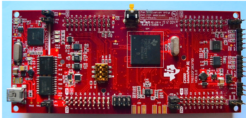
Figura 6.4: Vista superior del LaunchPad F28379D.
