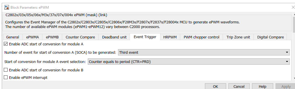
Figura 6.38: Configuración del inicio de ADC sincronizado con el ePWM.
