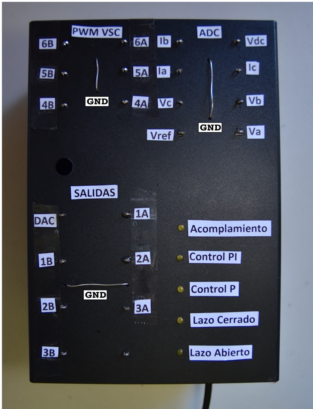
Figura 6.28: Encapsulado del VSC y Launchpad. Pines para osciloscopio.
