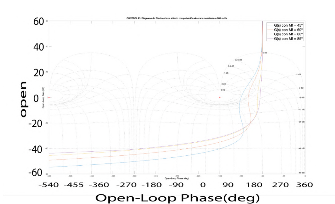
Figura 5.20: Respuesta en lazo abierto con pulsación de cruce constante con el control PI en tiempo continuo.
