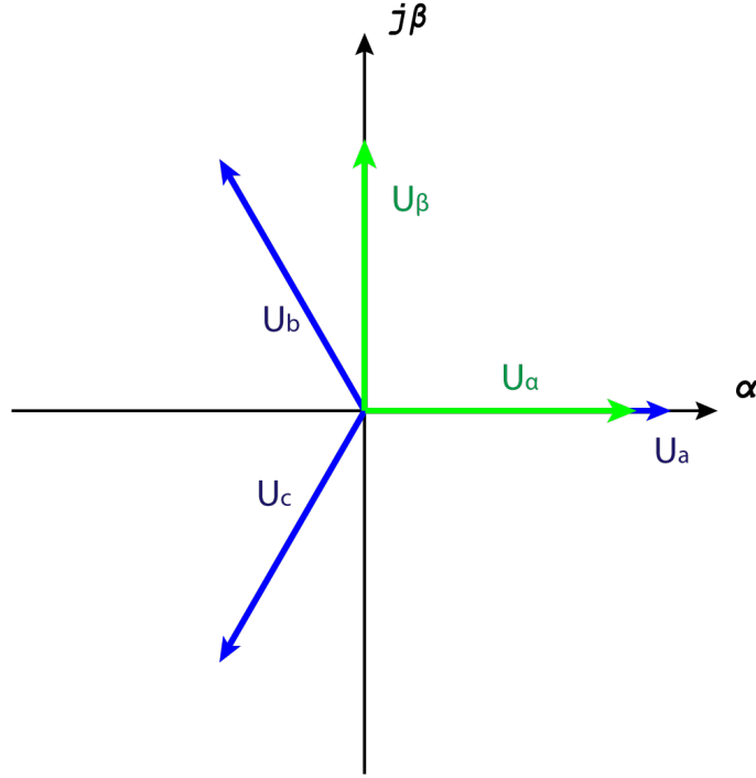
Figura 4.2: Transformada de Clarke.
