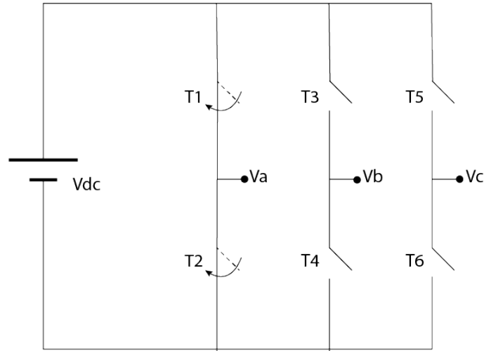
Figura 2.9: Hipotético cortocircuito de la fase A
