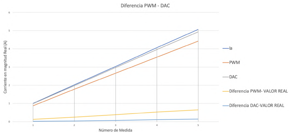
Figura 6.48: Diferencia en las medidas de PWM - DAC.
