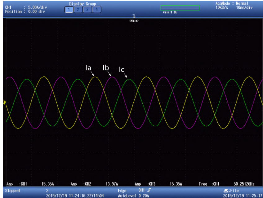
Figura 7.2: Corrientes trifásicas por las bobinas. La identificación de las señales se muestra en detalle en la figura. Ver Tabla 7.1.
