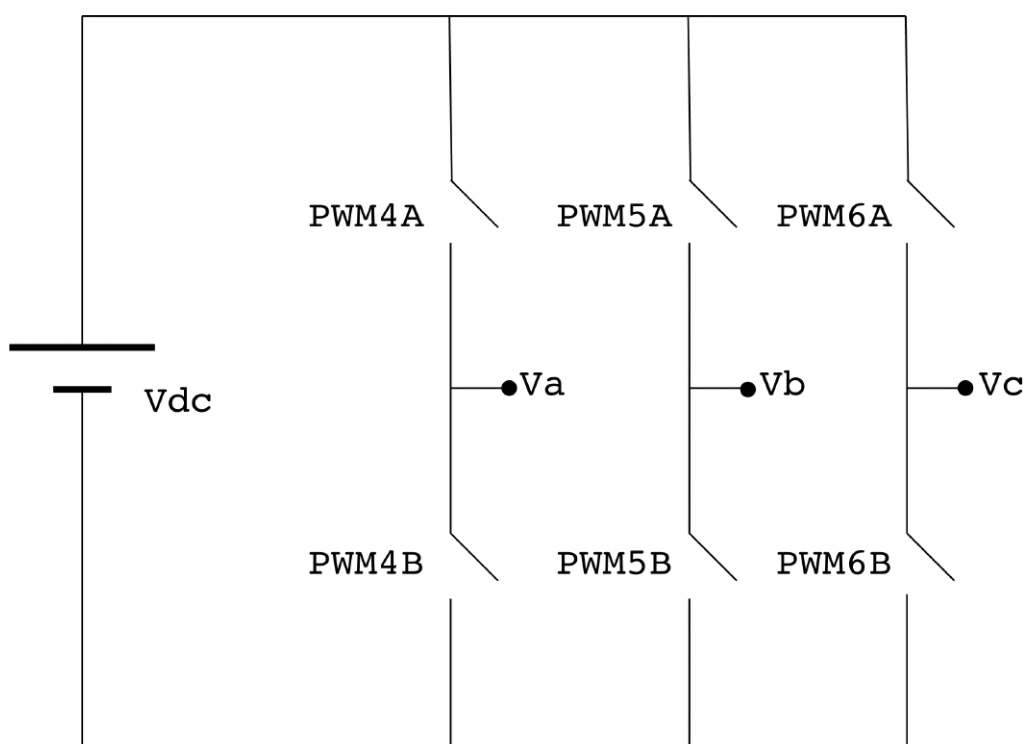
Figura 6.32: Diagrama de la nomenclatura de los PWM en Simulink para el VSC conectado al LaunchPad en su parte inferior (Sección 6.2.2).
