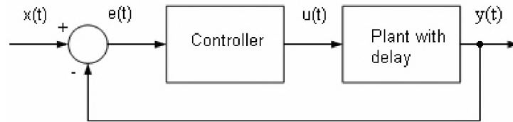
Figura 5.2: Diagrama de bloque de un control en tiempo continuo [41].
