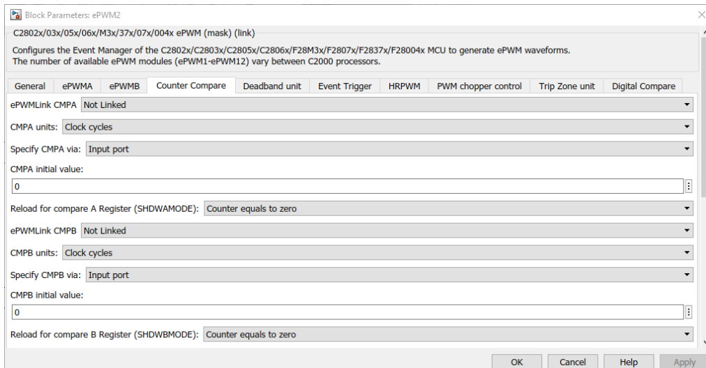
Figura 6.41: Configuración pestaña Counter Compare para obtención de señales por PWM. Contadores CMPA y CMPB .
