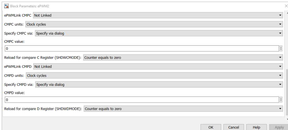
Figura 6.42: Configuración pestaña Counter Compare para obtención de señales por PWM. Contadores CMPC y CMPD .
