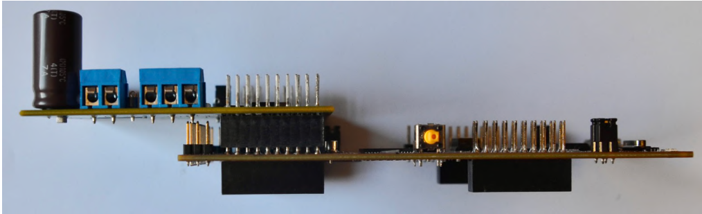
Figura 6.24: Conjunto LaunchPad con VSC con la conexión en la parte inferior. Vista lateral.
