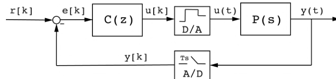
Figura 5.5: Diagrama de bloques de un control en tiempo discreto.
