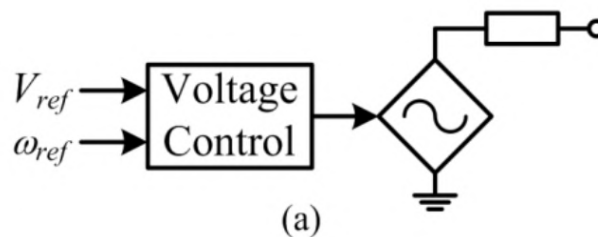
Figura 3.1: Diagrama de un convertidor en formato grid-forming [22].
