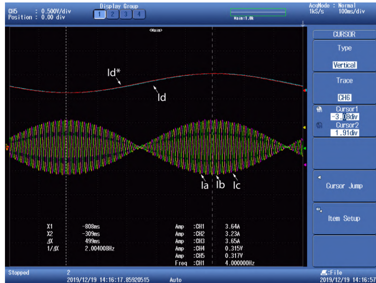
Figura 7.5: Corrientes trifásicas por las bobinas con referencia de eje corriente de eje d en forma senoidal de 4Hz. La identificación de las señales se muestran en detalle en la figura. Referencia de I_q = 0 .
