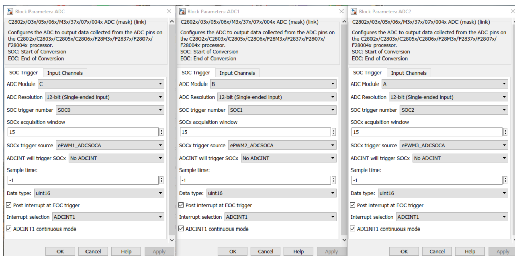
Figura 6.46: Configuración de los Bloque ADC.
