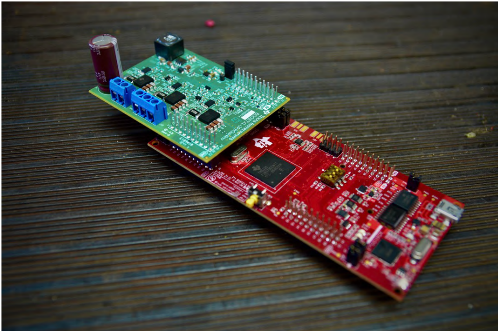
Figura 6.25: Conjunto LaunchPad con VSC con la conexión en la parte inferior. Vista en perspectiva.
