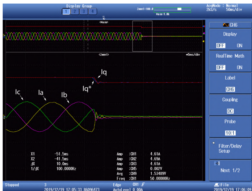
Figura 7.9: Corrientes trifásicas por las bobinas. Respuesta temporal de corriente de eje q. Referencia de I_d = 0 . La identificación de las señales se muestran en detalle en la figura.
