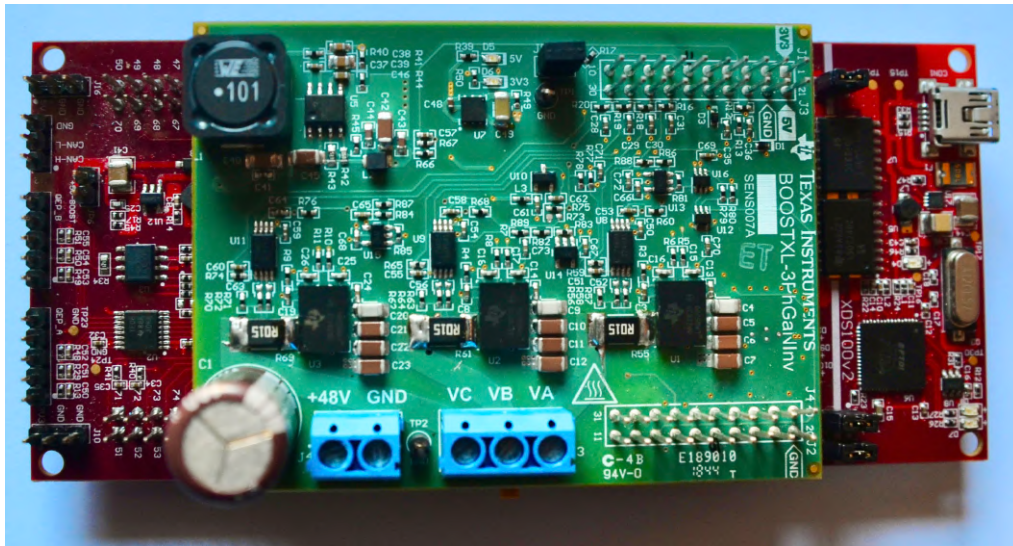
Figura 6.22: Conjunto LaunchPad con VSC con la conexión en la parte superior.
