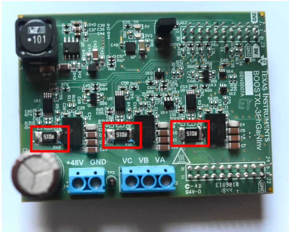
Figura 6.13: Vista superior del BOOSTXL-3PhGaNInv. Los recuadros son las resistencias cambiadas.
