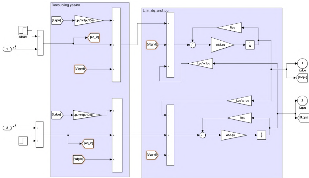
Figura 5.4: Simulink para la obtención de la planta en tiempo continuo.
