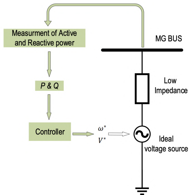
Figura 3.3: Diagrama de un convertidor en formato grid-supporting-forming con modelo de fuente de tensión [23].
