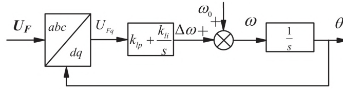
Figura 3.5: Diagrama de un bloque PLL [26].
