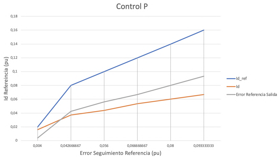
Figura 5.14: Gráfica de error de seguimiento de referencia de corriente de eje d con un Control P. Implantación hardware. Los datos del eje y están escalados a un 0.1 del valor en pu.
