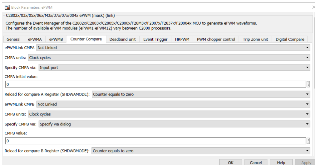
Figura 6.35: Configuración del Counter Compare .
