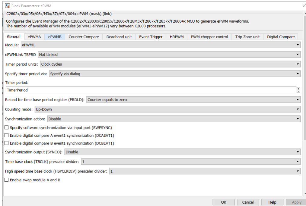
Figura 6.31: Bloque ePWM de Simulink. Librería TI C2000.
