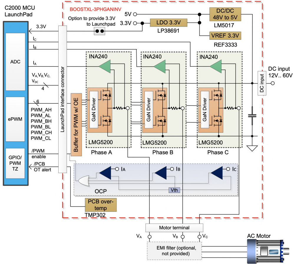
Figura 6.15: Diagrama funcional del BOOSTXL-3PhGaNInv [47].
