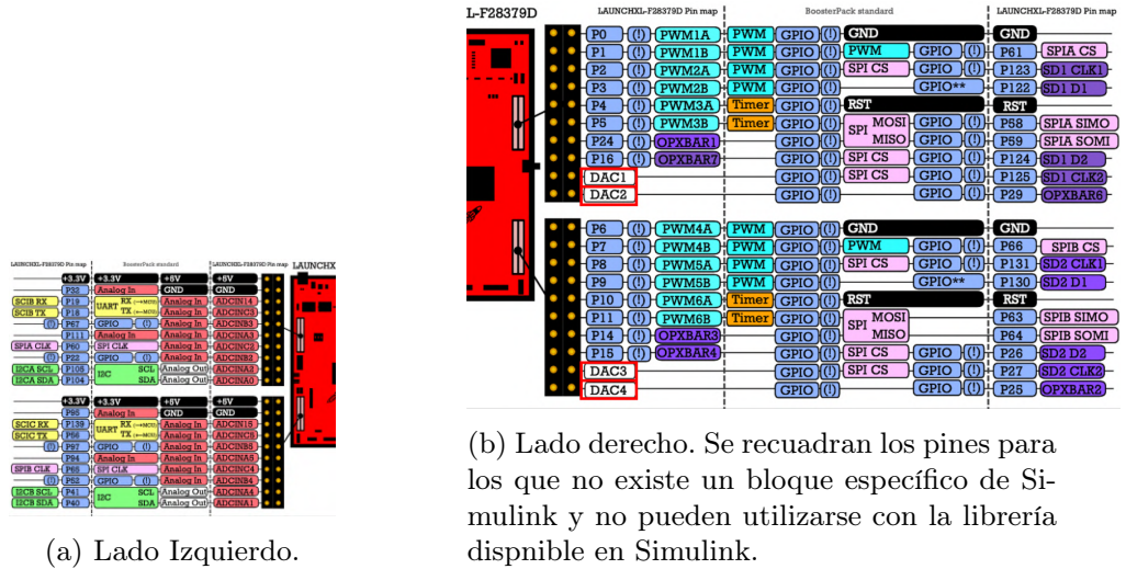
Figura 5: Vista de detalle del Pinout de la tarjeta LAUNCHXL - F28379D. [2].
