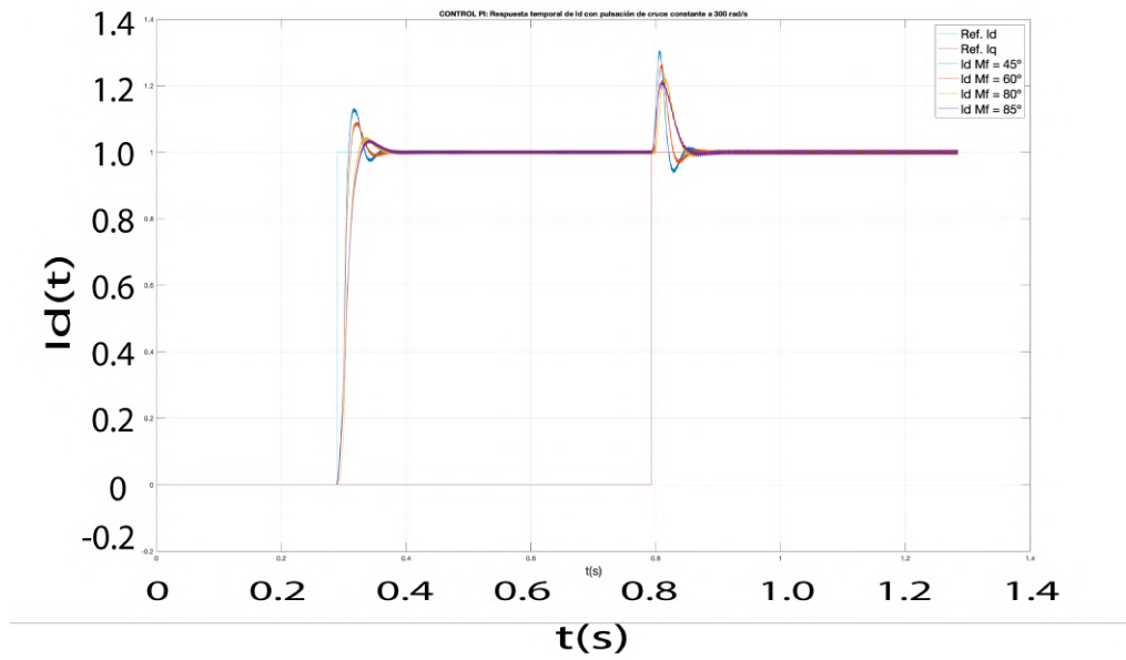
Figura 5.17: Respuesta temporal de I_d con pulsación de cruce constante con el control PI en tiempo continuo. Pulso de I_d = 1 en 0.3s. Pulso de I_q = 1 en 0.8s.
