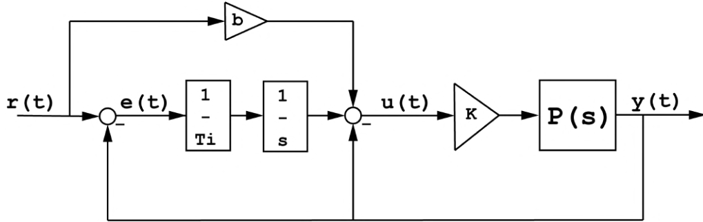
Figura 5.3: Diagrama de bloques de un control PI en formato paralelo.
