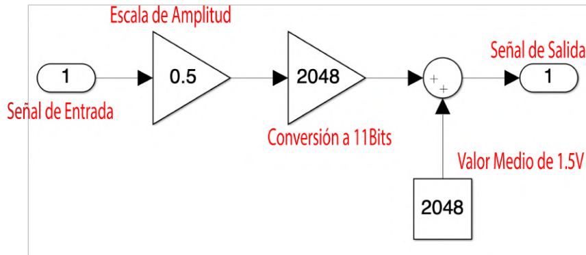
Figura 6.50: Diagrama de bloques para obtener una señal por el DAC o PWM. El valor medio de 1.5V real podría variar.
