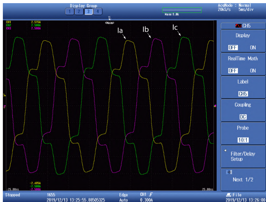
Figura 7.3: Corrientes trifásicas por las bobinas saturadas.
