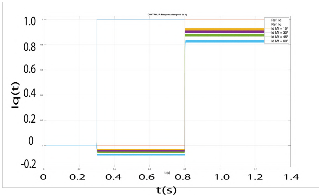
Figura 5.10: Respuesta temporal de eje q de un Control P en tiempo continuo. Pulso de I_d = 1 en 0.3s. Pulso de I_q = 1 en 0.8s.
