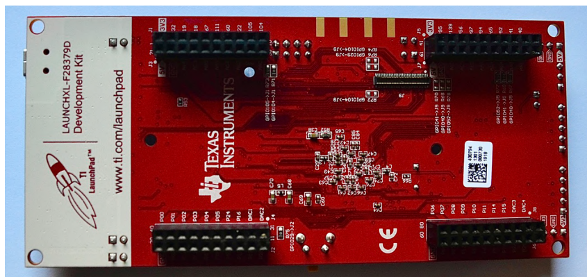
Figura 6.5: Vista inferior del LaunchPad F28379D.
