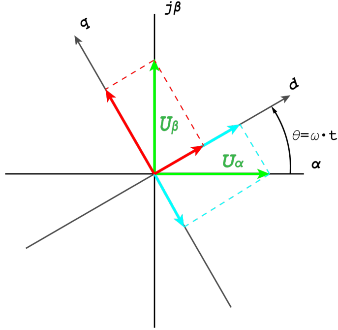
Figura 4.3: Transformada de Park.
