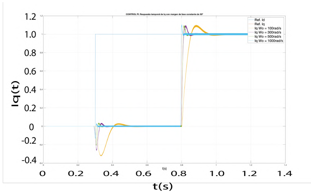
Figura 5.16: Respuesta temporal de I_q con margen de fase constant con el control PI en tiempo continuo. Pulso de I_d = 1 en 0.3s. Pulso de I_q = 1 en 0.8s.
