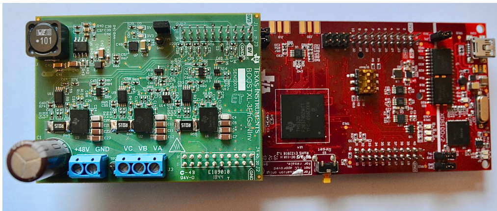
Figura 6.23: Conjunto LaunchPad con VSC con la conexión en la parte inferior.
