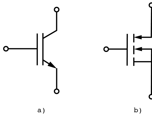
Figura 2.7: Diagrama de un IGBT como a) BJT b) MOSFET
