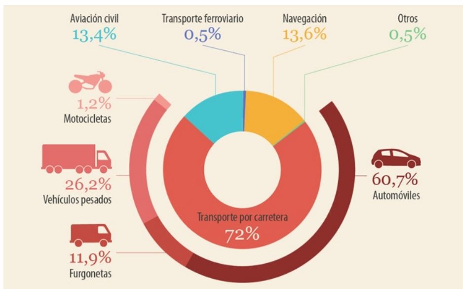
Figura 3: Emisiones de CO2 por medio de transporte en la UE
