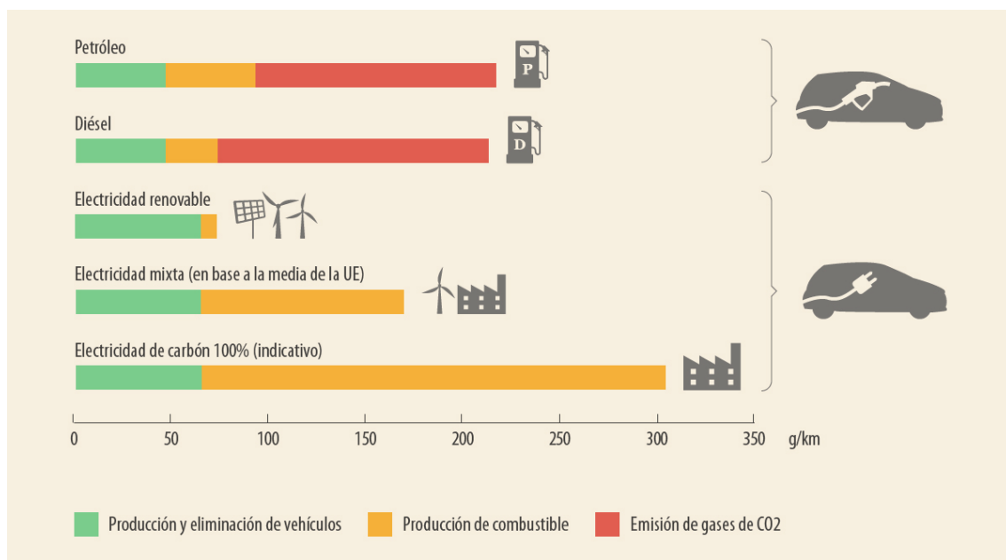
Figura 5: Ciclo de vida de las emisiones de CO 2 originadas para distintos tipos de vehículos y tipos de combustible en la UE
