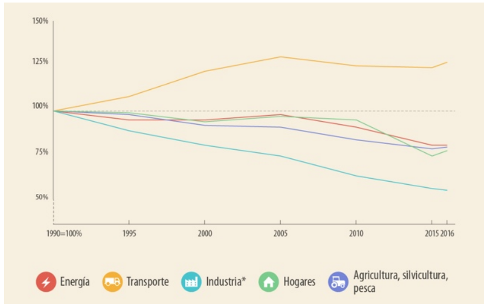
Figura 2: Evolución de las emisiones de CO2 en la UE por sector
