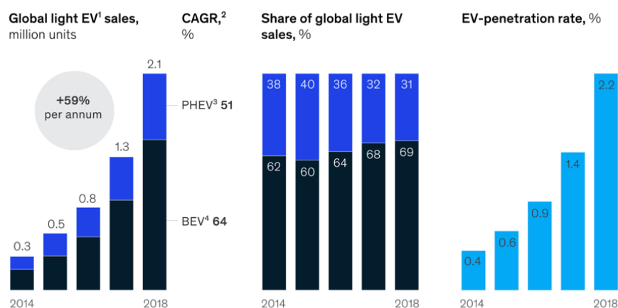
Figura 4: Ventas a nivel global de los vehículos eléctricos
