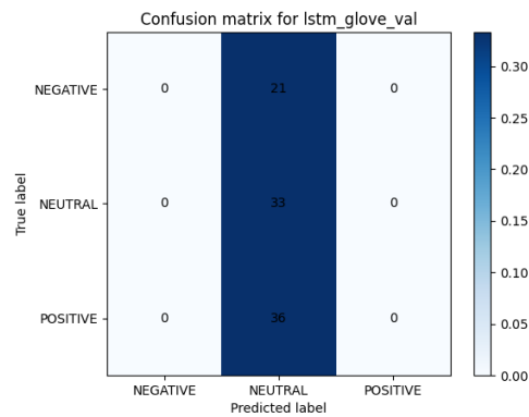
Figura 105: Matriz de confusión del modelo LSTM con GLOVE
