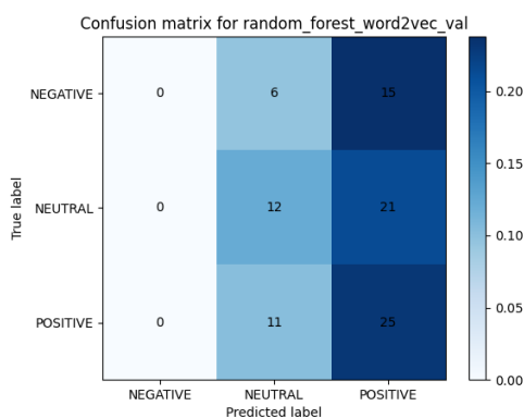
Figura 90: Matriz de confusión del modelo Random Forest con Word2Vec
