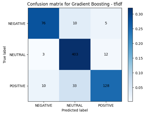
Figura 40: Matriz de confusión del modelo Gradient Boosting con TF-IDF
