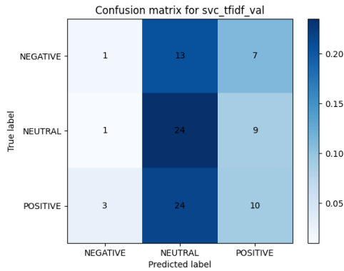
Figura 94: Matriz de confusión del modelo SVM con TF-IDF
