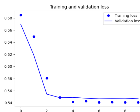
Figura 69: Curva de loss del modelo LSTM con GLOVE
