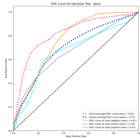
Figura 39: Curva ROC del modelo Decission Tree con GLOVE
