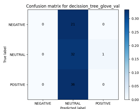
Figura 80: Matriz de confusión del modelo Decision Tree con GLOVE
