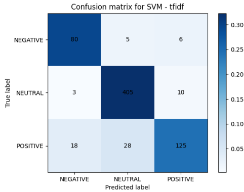
Figura 52: Matriz de confusión del modelo SVM con TF-IDF
