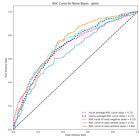
Figura 33: Curva ROC del modelo Naive Bayes con GLOVE
