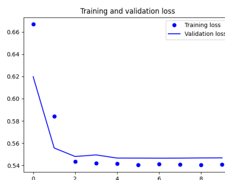
Figura 65: Curva de loss del modelo LSTM con TF-IDF
