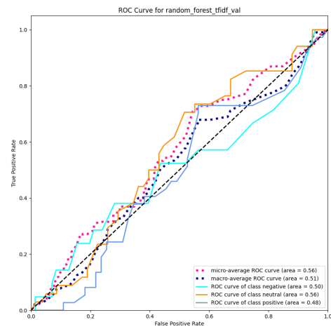
Figura 89: Curva ROC del modelo Random Forest con TF-IDF
