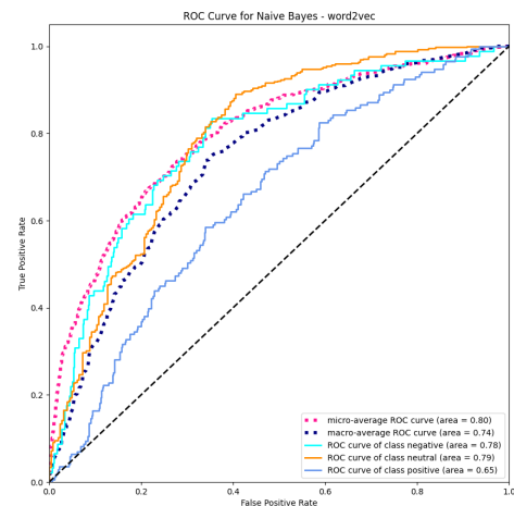
Figura 31: Curva ROC del modelo Naive Bayes con Word2Vec
