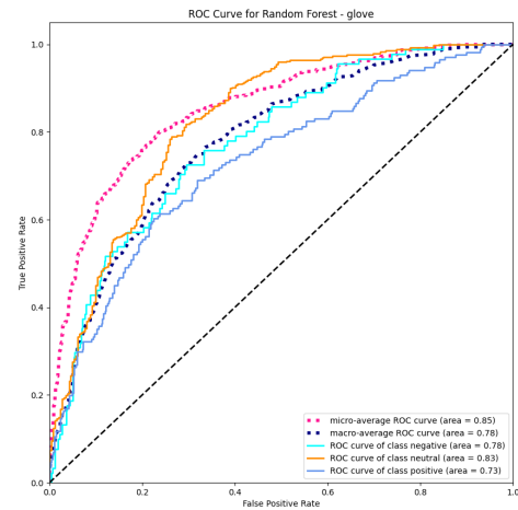
Figura 51: Curva ROC del modelo Random Forest con GLOVE
