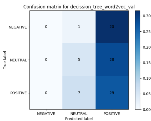
Figura 78: Matriz de confusión del modelo Decission Tree con Word2Vec
