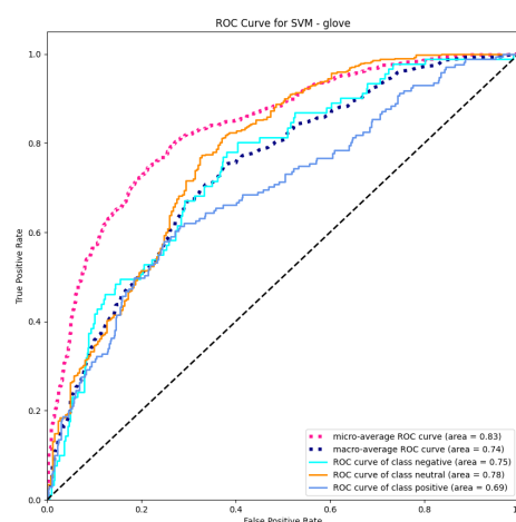
Figura 57: Curva ROC del modelo SVM con GLOVE
