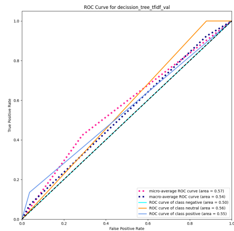
Figura 77: Curva ROC del modelo Decission Tree con TF-IDF
