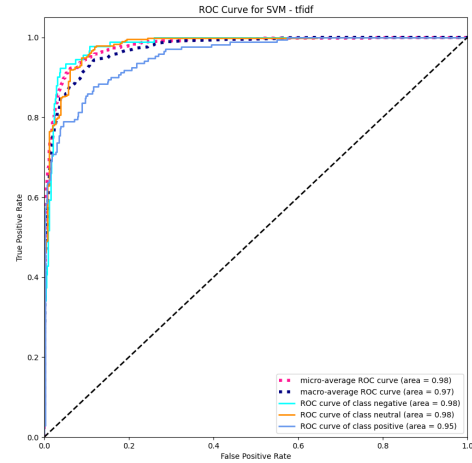
Figura 53: Curva ROC del modelo SVM con TF-IDF
