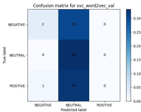
Figura 96: Matriz de confusión del modelo SVM con Word2Vec
