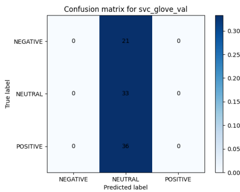
Figura 98: Matriz de confusión del modelo SVM con GLOVE
