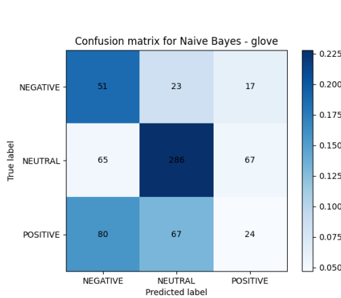
Figura 32: Matriz de confusión del modelo Naive Bayes con GLOVE
