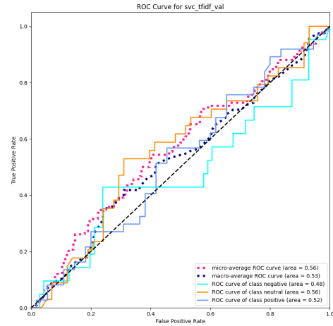
Figura 95: Curva ROC del modelo SVM con TF-IDF
