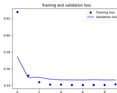
Figura 63: Curva de loss del modelo RNN con GLOVE
