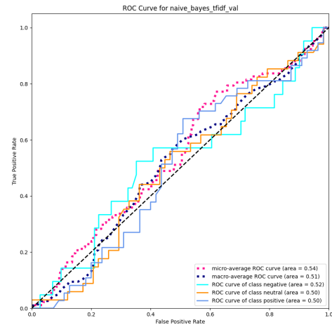
Figura 71: Curva ROC del modelo Naive Bayes con TF-IDF
