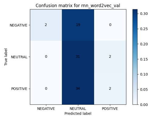
Figura 101: Matriz de confusión del modelo RNN con Word2Vec
