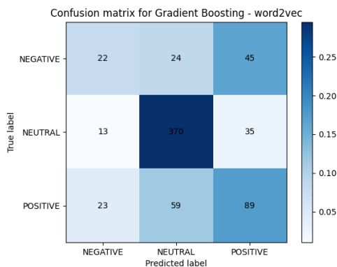
Figura 42: Matriz de confusión del modelo Gradient Boosting con Word2Vec
