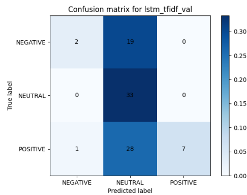
Figura 103: Matriz de confusión del modelo LSTM con TF-IDF
