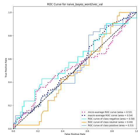
Figura 73: Curva ROC del modelo Naive Bayes con Word2Vec
