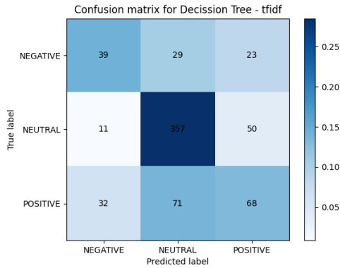
Figura 34: Matriz de confusión del modelo Decission Tree con TF-IDF
