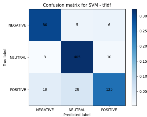
Figura 23: Matriz de confusión del modelo SVM con TF-IDF
