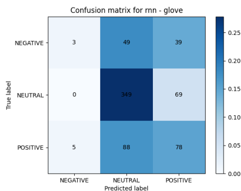
Figura 62: Matriz de confusión del modelo RNN con GLOVE
