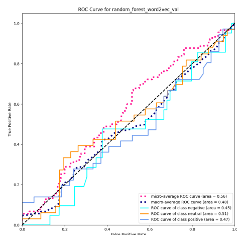
Figura 91: Curva ROC del modelo Random Forest con Word2Vec
