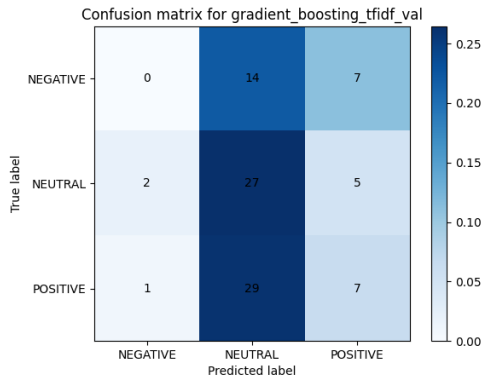
Figura 82: Matriz de confusión del modelo Gradient Boosting con TF-IDF
