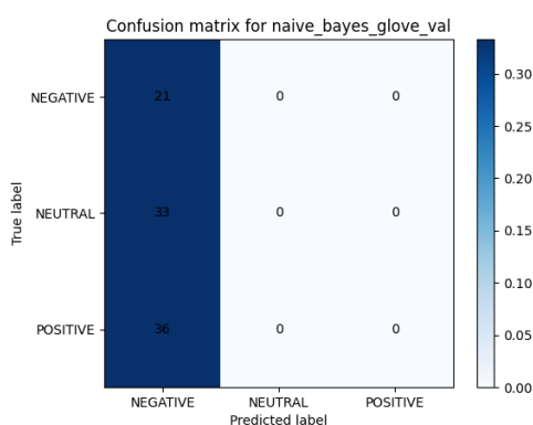
Figura 74: Matriz de confusión del modelo Naive Bayes con GLOVE
