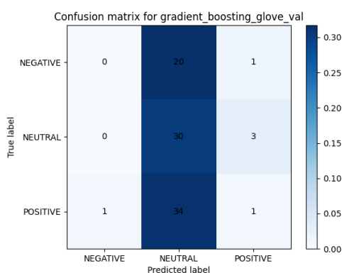
Figura 86: Matriz de confusión del modelo Gradient Boosting con GLOVE
