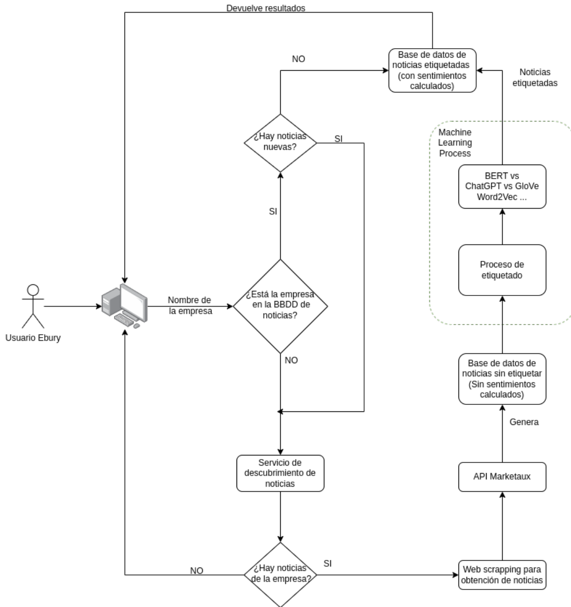
Figura 3: Diagrama de flujo detallado
