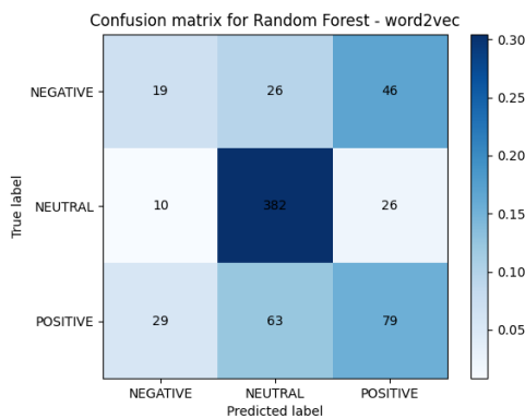
Figura 48: Matriz de confusión del modelo Random Forest con Word2Vec
