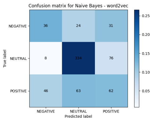
Figura 30: Matriz de confusión del modelo Naive Bayes con Word2Vec
