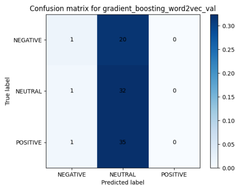
Figura 84: Matriz de confusión del modelo Gradient Boosting con Word2Vec
