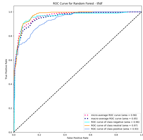
Figura 47: Curva ROC del modelo Random Forest con TF-IDF
