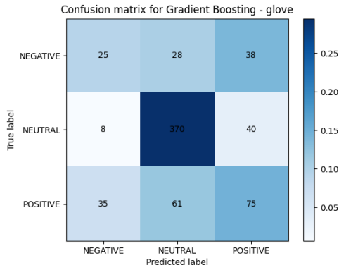
Figura 44: Matriz de confusión del modelo Gradient Boosting con GLOVE
