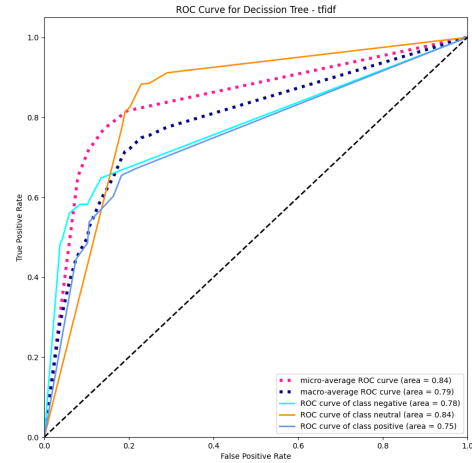
Figura 35: Curva ROC del modelo Decission Tree con TF-IDF
