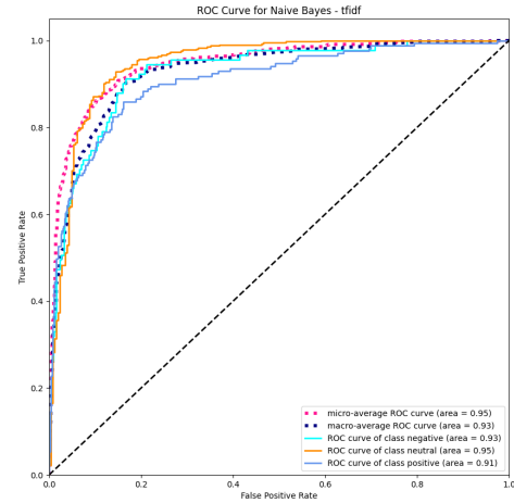
Figura 29: Curva ROC del modelo Naive Bayes con TF-IDF
