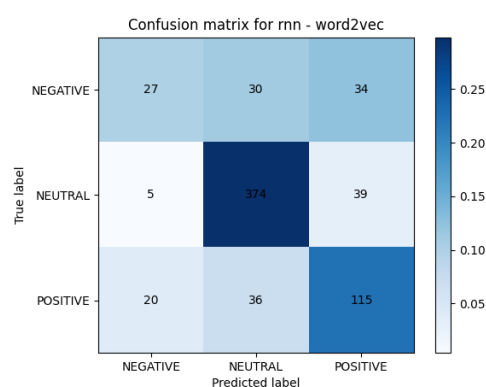
Figura 60: Matriz de confusión del modelo RNN con Word2Vec
