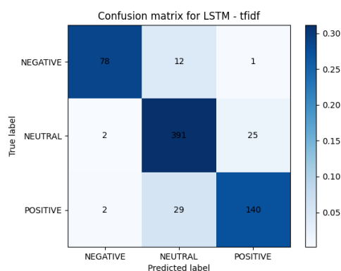
Figura 64: Matriz de confusión del modelo LSTM con TF-IDF
