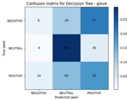
Figura 38: Matriz de confusión del modelo Decission Tree con GLOVE
