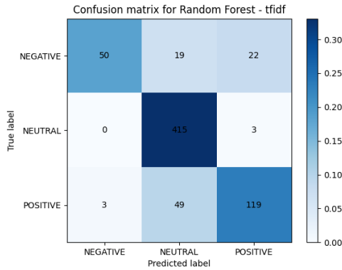
Figura 46: Matriz de confusión del modelo Random Forest con TF-IDF
