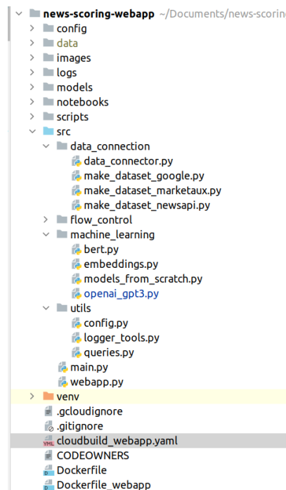
Figura 22: Estructura de código del proyecto
