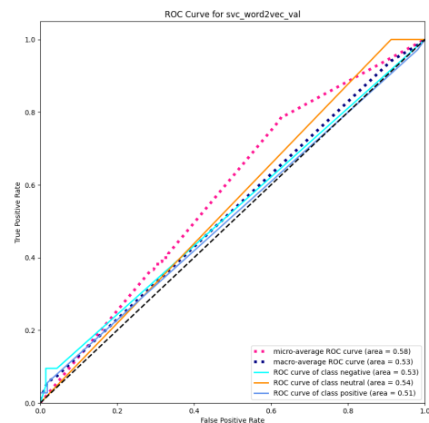
Figura 97: Curva ROC del modelo SVM con Word2Vec
