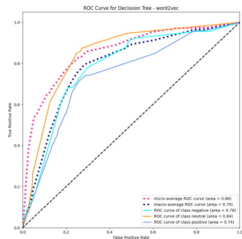
Figura 37: Curva ROC del modelo Decission Tree con Word2Vec
