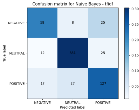
Figura 28: Matriz de confusión del modelo Naive Bayes con TF-IDF
