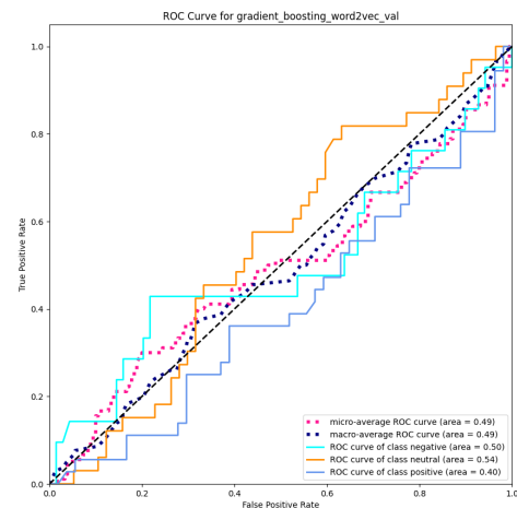
Figura 85: Curva ROC del modelo Gradient Boosting con Word2Vec
