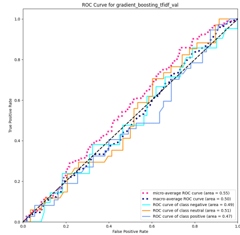
Figura 83: Curva ROC del modelo Gradient Boosting con TF-IDF
