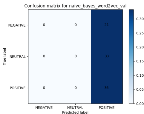
Figura 72: Matriz de confusión del modelo Naive Bayes con Word2Vec
