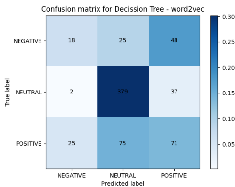
Figura 36: Matriz de confusión del modelo Decission Tree con Word2Vec
