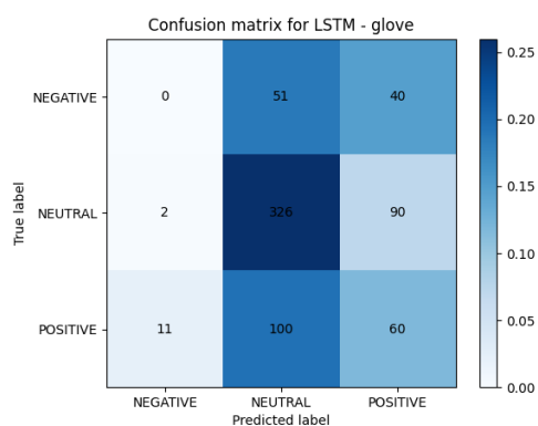
Figura 68: Matriz de confusión del modelo LSTM con GLOVE
