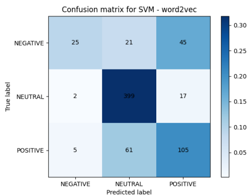
Figura 54: Matriz de confusión del modelo SVM con Word2Vec
