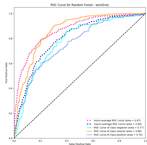
Figura 49: Curva ROC del modelo Random Forest con Word2Vec
