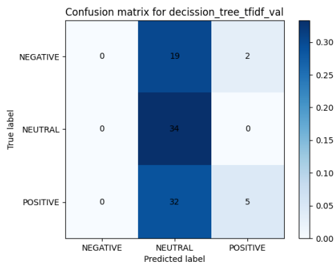
Figura 76: Matriz de confusión del modelo Decission Tree con TF-IDF
