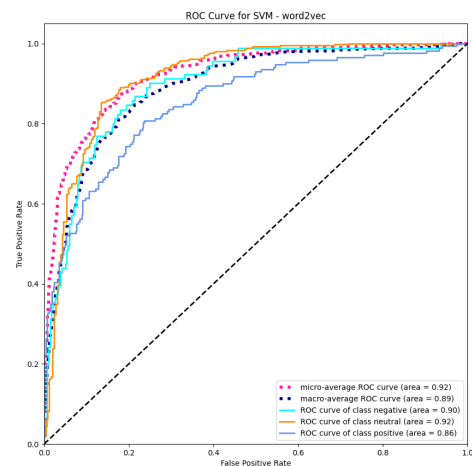
Figura 55: Curva ROC del modelo SVM con Word2Vec
