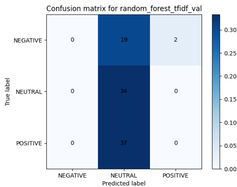
Figura 88: Matriz de confusión del modelo Random Forest con TF-IDF
