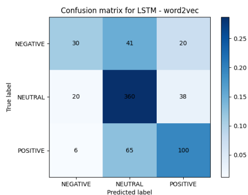
Figura 66: Matriz de confusión del modelo LSTM con Word2Vec
