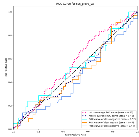
Figura 99: Curva ROC del modelo SVM con GLOVE
