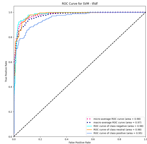
Figura 24: Curva ROC del modelo SVM con TF-IDF
