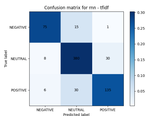
Figura 58: Matriz de confusión del modelo RNN con TF-IDF
