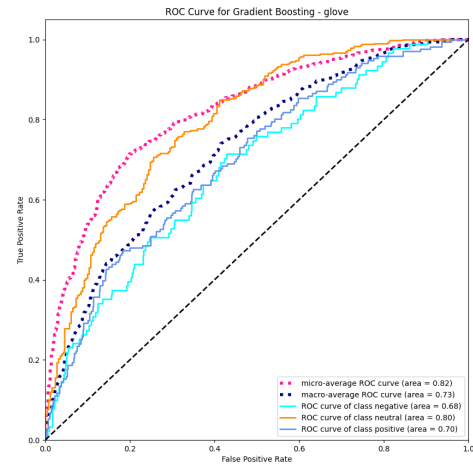
Figura 45: Curva ROC del modelo Gradient Boosting con GLOVE
