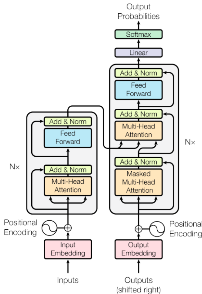
Figura 1: Arquitectura de un Transformer. Encoder y Decoder.
