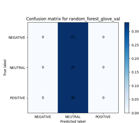
Figura 92: Matriz de confusión del modelo Random Forest con GLOVE
