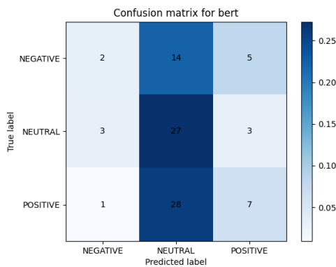
Figura 25: Matriz de confusión del modelo FinancialBert
