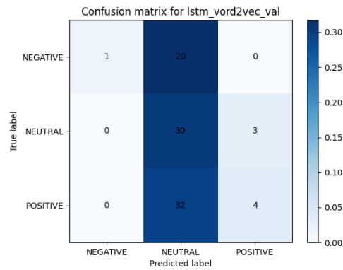
Figura 104: Matriz de confusión del modelo LSTM con Word2Vec
