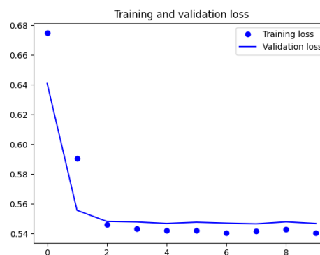
Figura 67: Curva de loss del modelo LSTM con Word2Vec
