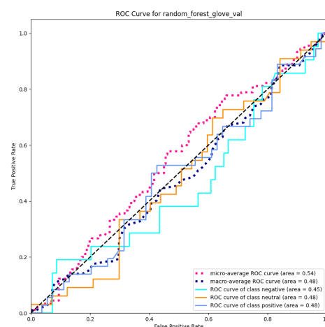
Figura 93: Curva ROC del modelo Random Forest con GLOVE
