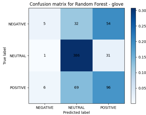
Figura 50: Matriz de confusión del modelo Random Forest con GLOVE
