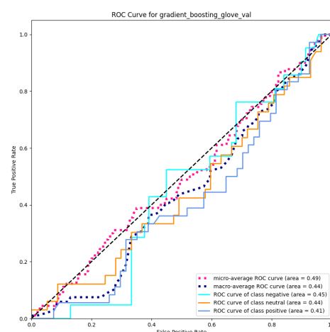
Figura 87: Curva ROC del modelo Gradient Boosting con GLOVE
