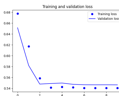
Figura 59: Curva de loss del modelo RNN con TF-IDF
