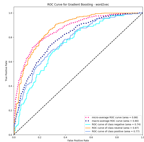
Figura 43: Curva ROC del modelo Gradient Boosting con Word2Vec
