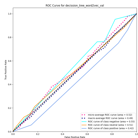
Figura 79: Curva ROC del modelo Decission Tree con Word2Vec
