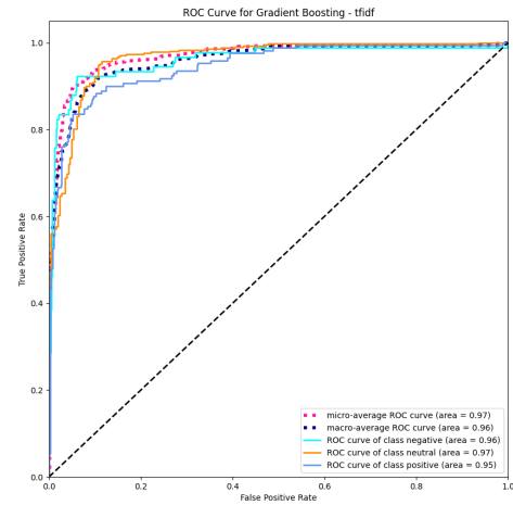
Figura 41: Curva ROC del modelo Gradient Boosting con TF-IDF
