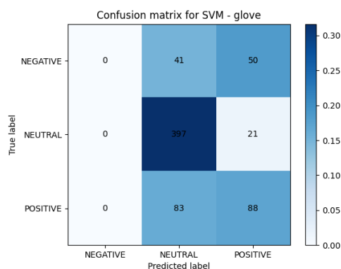
Figura 56: Matriz de confusión del modelo SVM con GLOVE
