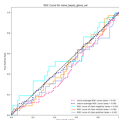
Figura 75: Curva ROC del modelo Naive Bayes con GLOVE
