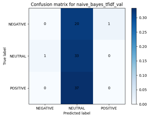
Figura 70: Matriz de confusión del modelo Naive Bayes con TF-IDF
