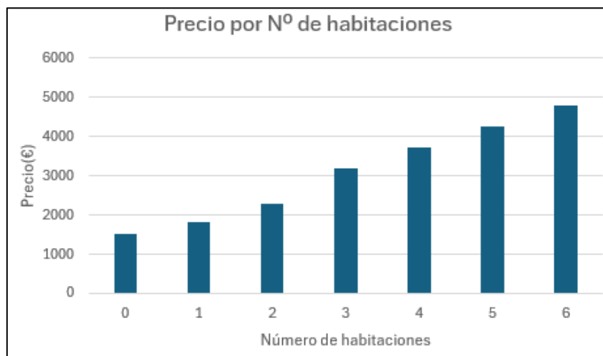
Ilustración 8: Precio medio de alquiler por número de habitaciones
