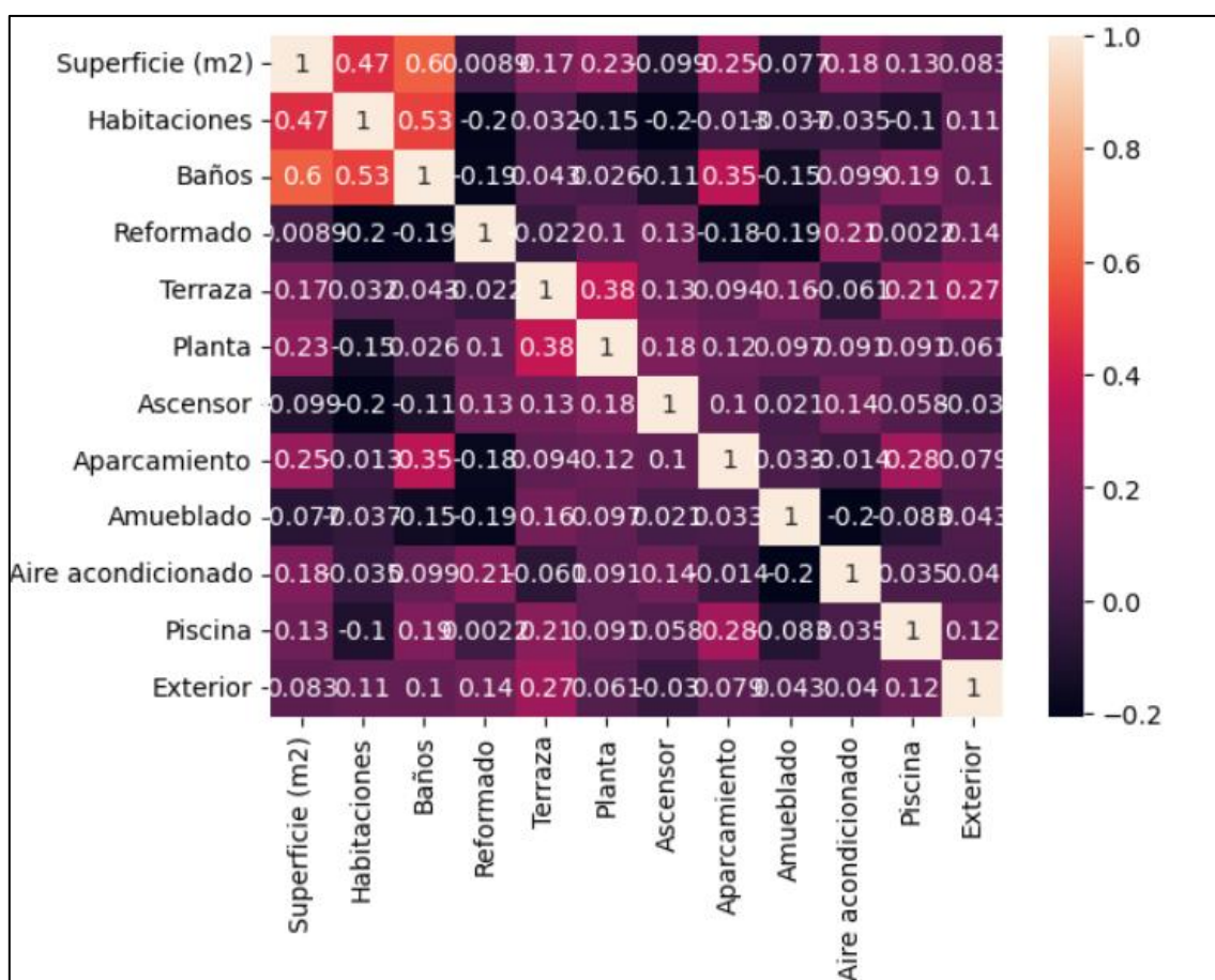
Ilustración 22: Matriz correlación modelo propiedades en venta (datos recogidos a mano) Precio > 1,000,000€
