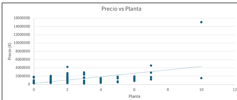
Ilustración 9: Dispersión de precio de venta según la planta
