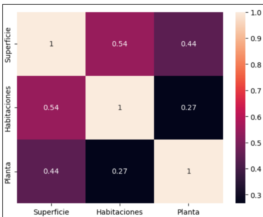
Ilustración 26: Matriz de correlación modelo final propiedades en venta (vía API)
