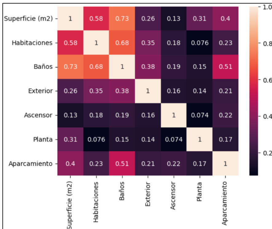
Ilustración 28: Matriz correlación modelo propiedades en venta (vía API y datos recogidos a mano)
