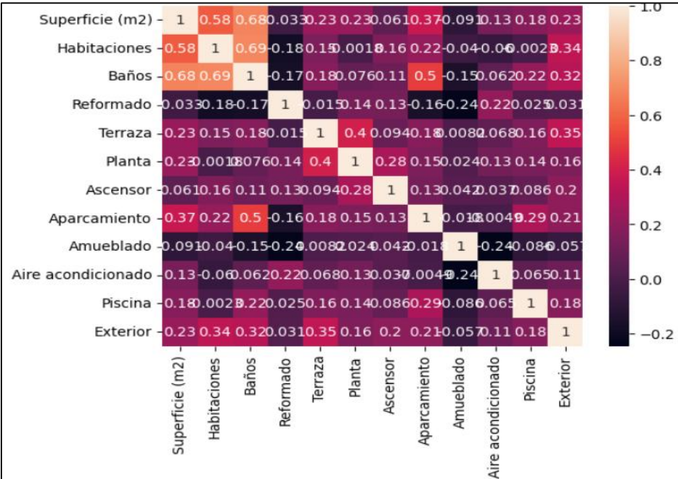
Ilustración 11: Matriz de correlación
