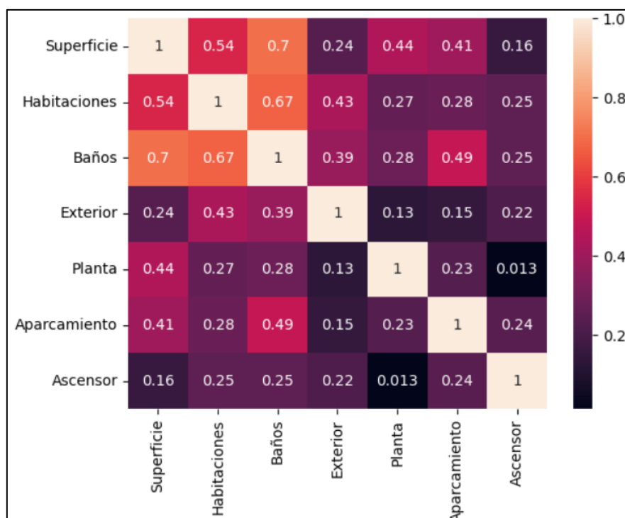
Ilustración 4: Matriz de correlación propiedades en venta (vía API)
