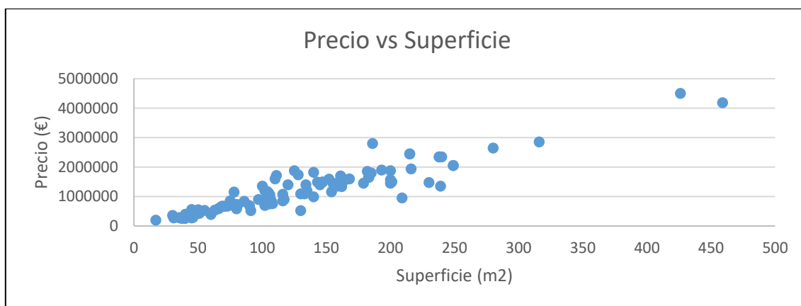
Ilustración 5: Relación entre precio de venta y superficie de la vivienda en Nuevos Ministerios–Ríos Rosas
