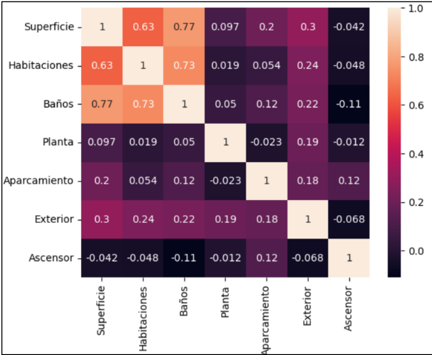
Ilustración 3: Matriz de correlación propiedades en alquiler
