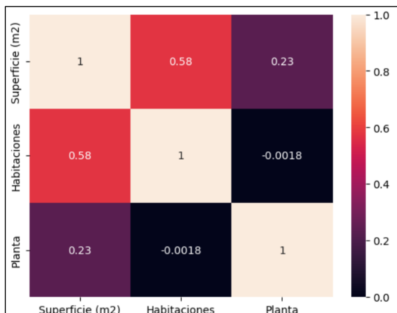
Ilustración 19: Matriz de correlación modelo final de propiedades en venta (datos recogidos a mano)
