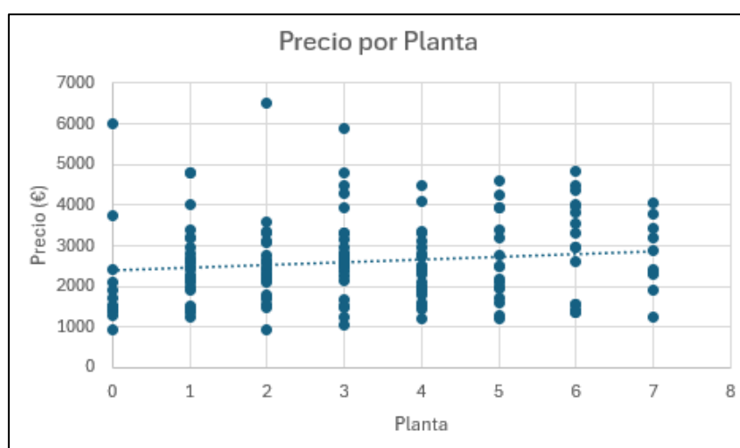
Ilustración 10: Dispersión de precio de alquiler según la planta
