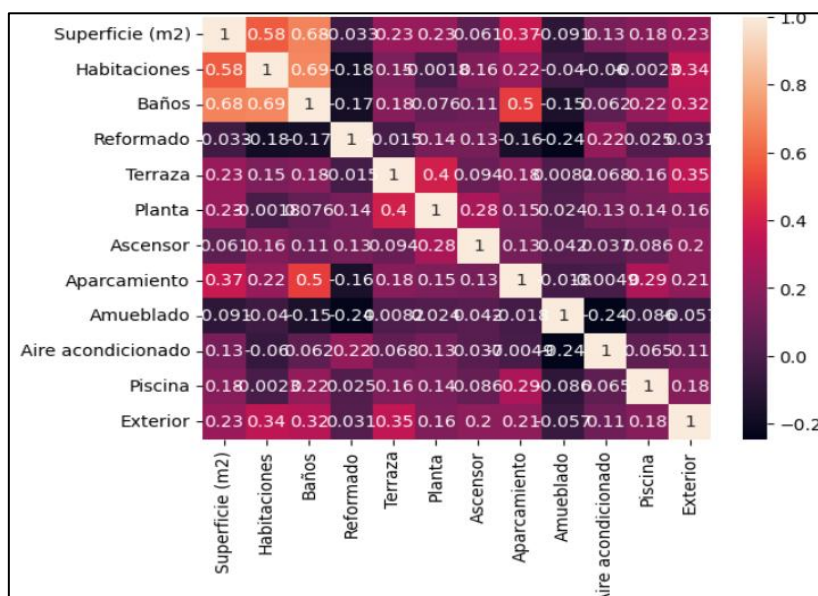
Ilustración I: Matriz de correlación
