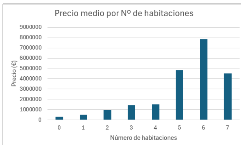
Ilustración 7: Precio medio de venta por número de habitaciones
