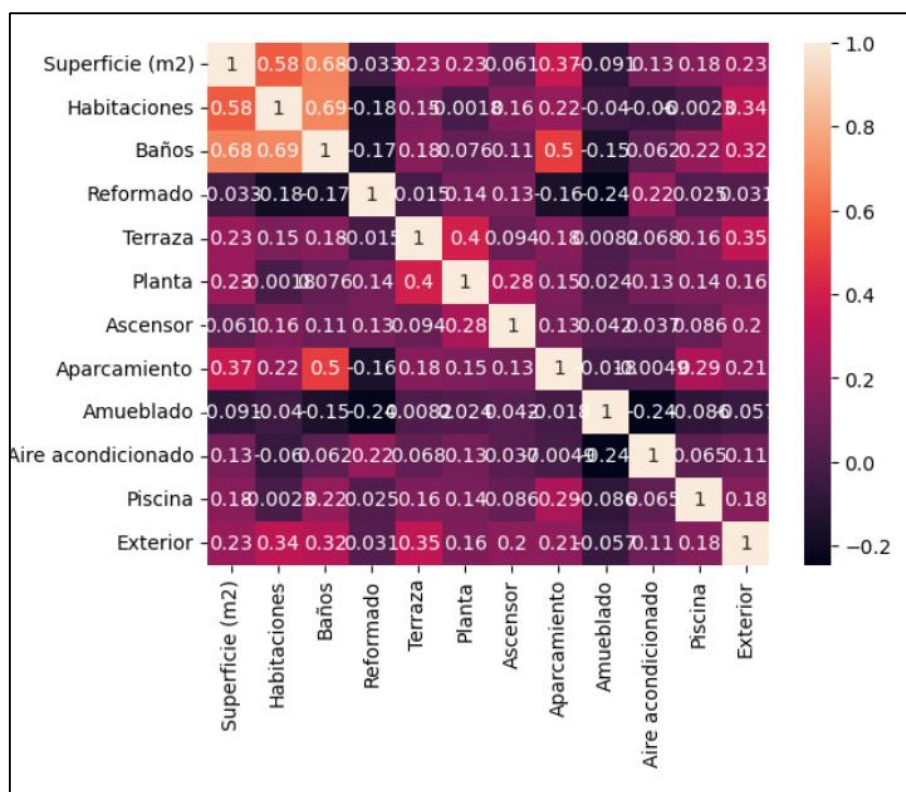
Ilustración 21: Matriz correlación modelo ventas (datos recogidos a mano) superficie > 100 m²
