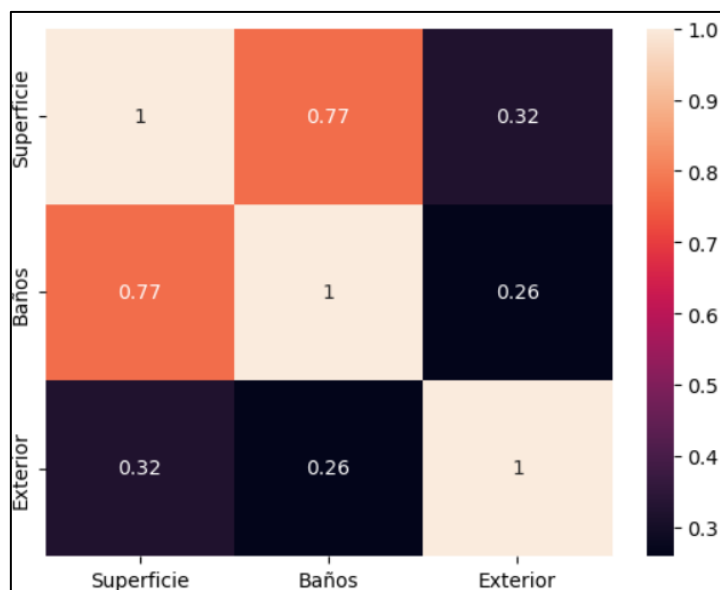
Ilustración 24: Matriz correlación modelo final propiedades en alquiler
