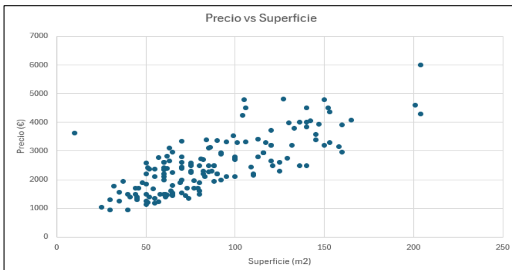
Ilustración 6: Relación entre precio de alquiler y superficie de la vivienda
