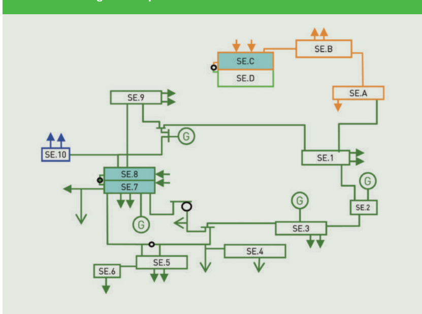
Figura 1. Esquema unifilar de la red de alta tensión
