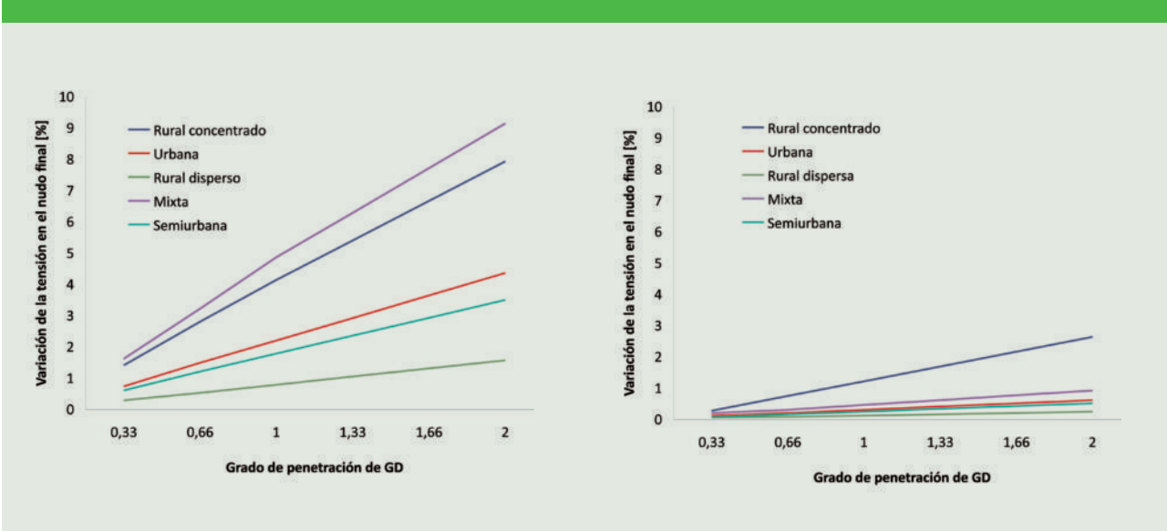
Figura 6. Variación de la tensión en función del grado de penetración en horas punta (izq.) y valle (dcha.)
