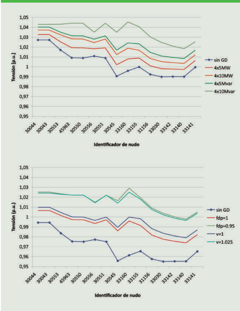
Figura 5. Variación de la tensión en función de la inyección de P y Q de GD (arriba) y con diferentes estrategias de control (abajo)
