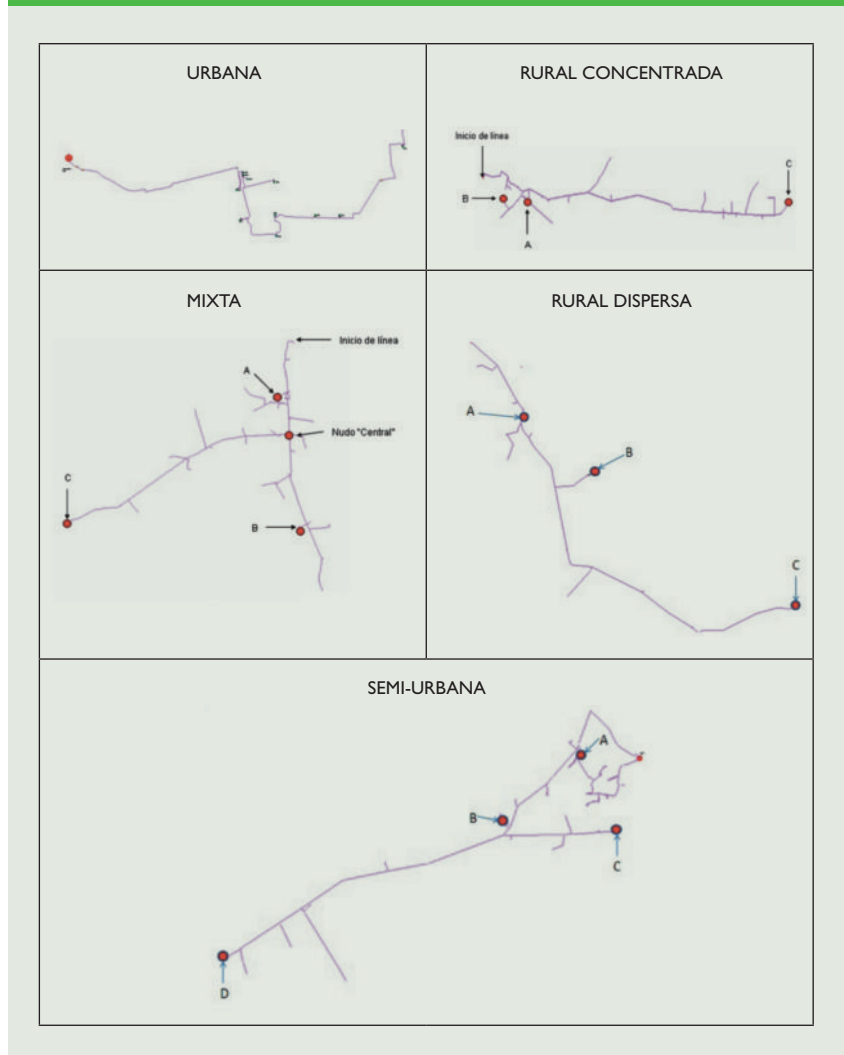
Figura 2. Esquemas unifilares de las redes de media tensión
