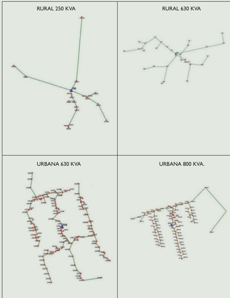
Figura 3. Esquemas unifilares de las redes de baja tensión
