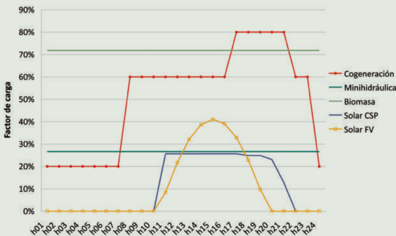
Figura 4. Perfil típico de generación de las distintas tecnologías renovables y cogeneración
