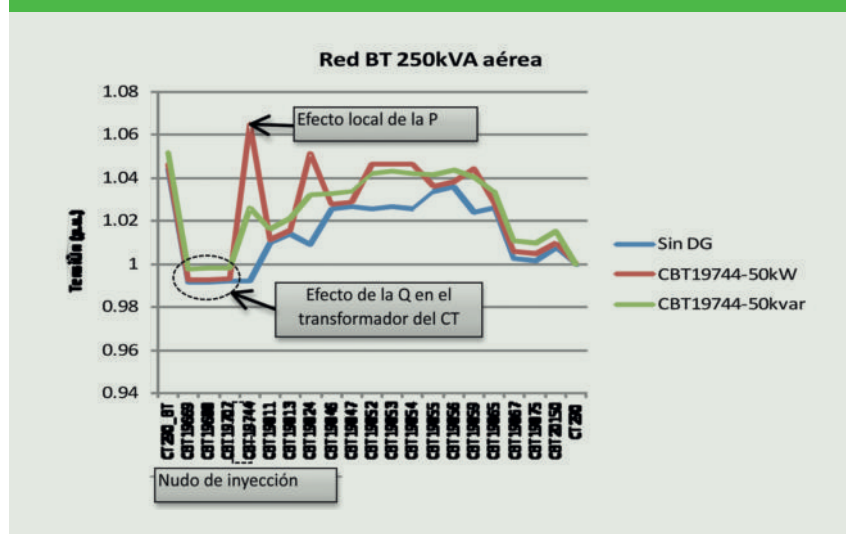
Figura 8. Variación de la tensión en función de la potencia inyectada a final de línea
