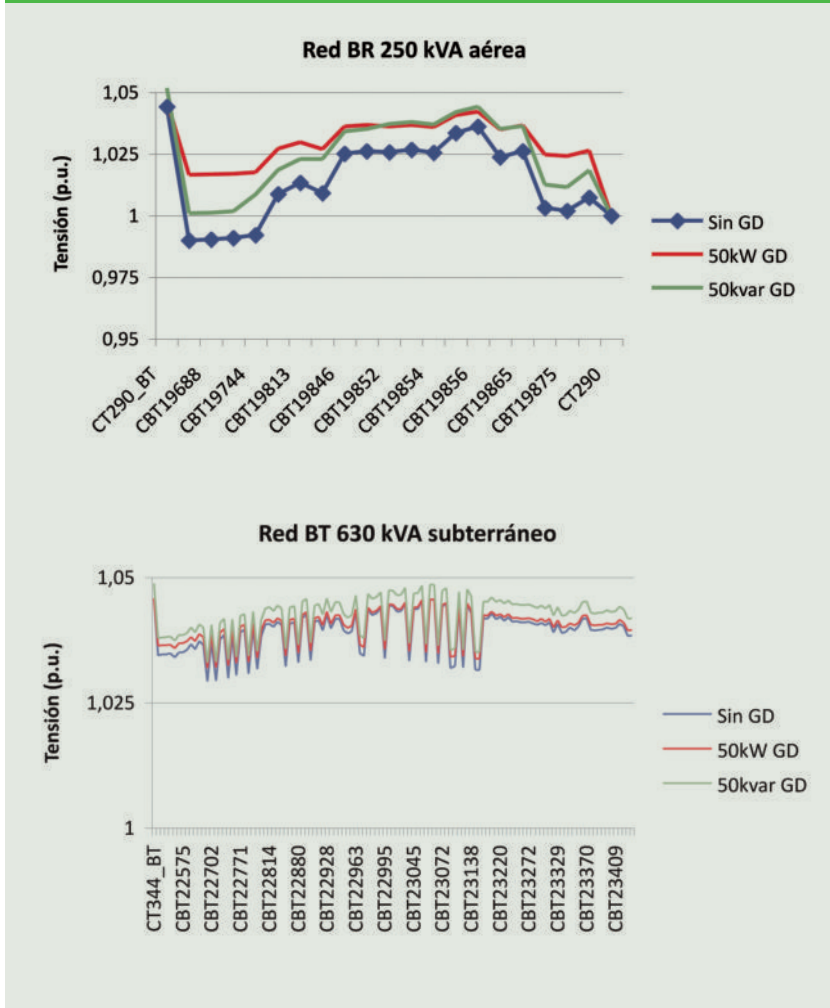
Figura 9. Variación de la tensión en función de la potencia inyectada
