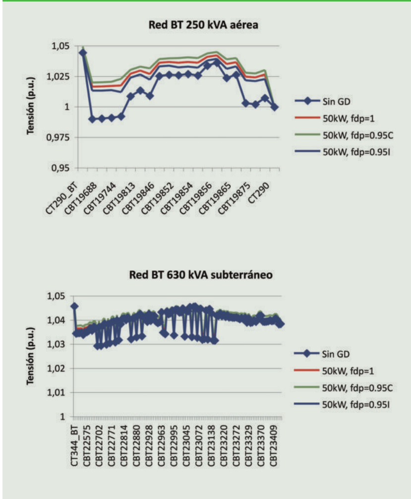
Figura 12. Variación de la tensión en función de la estrategia de control de tensión
