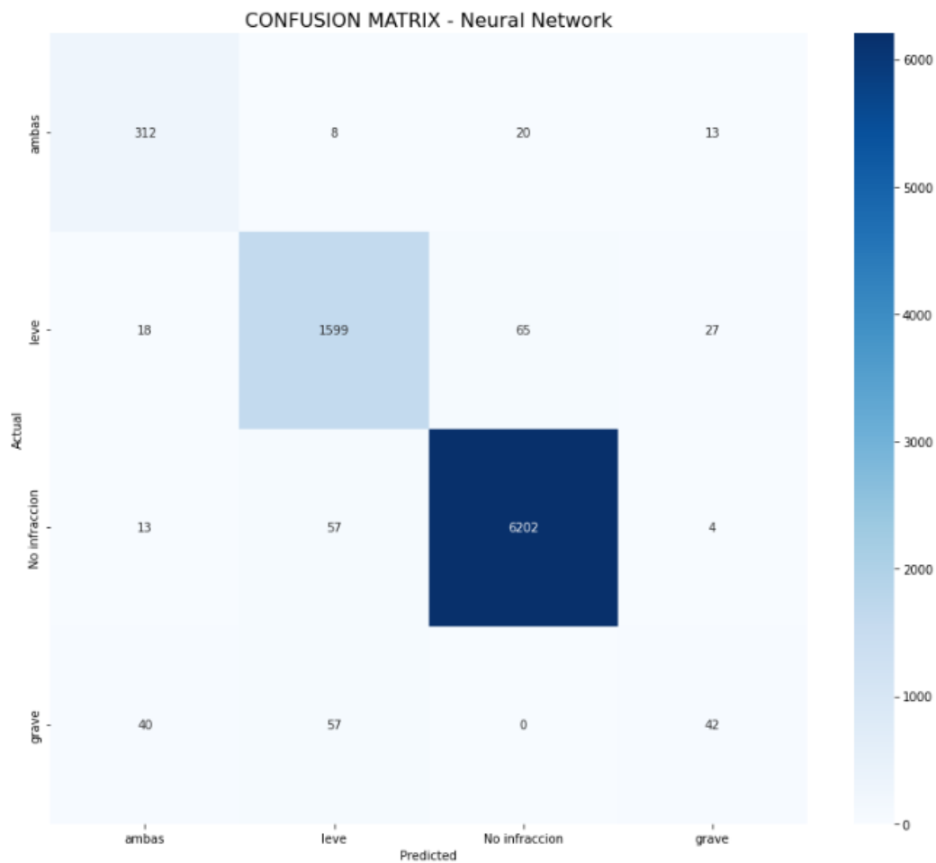
Ilustración 15. Matriz de Confusión para el modelo de Redes Neuronales
