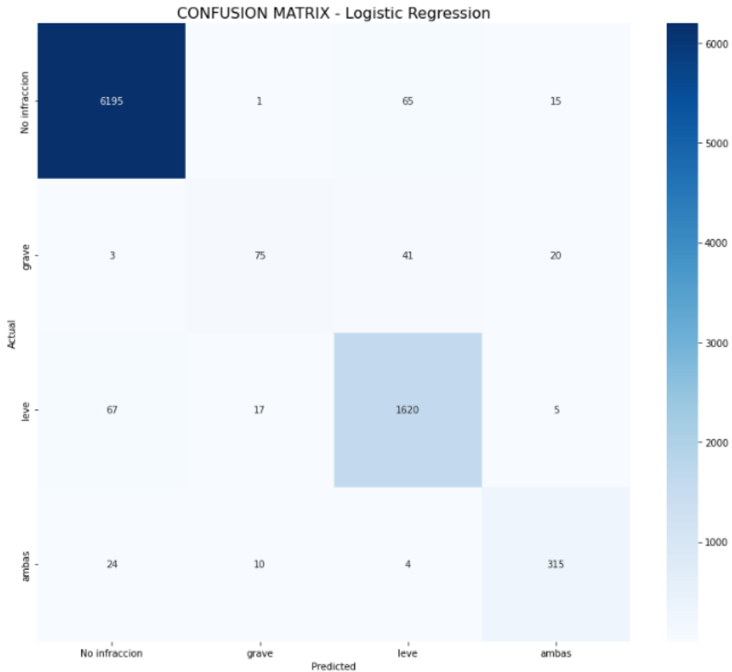
Ilustración 14. Matriz de Confusión para el modelo de Regresión Logística
