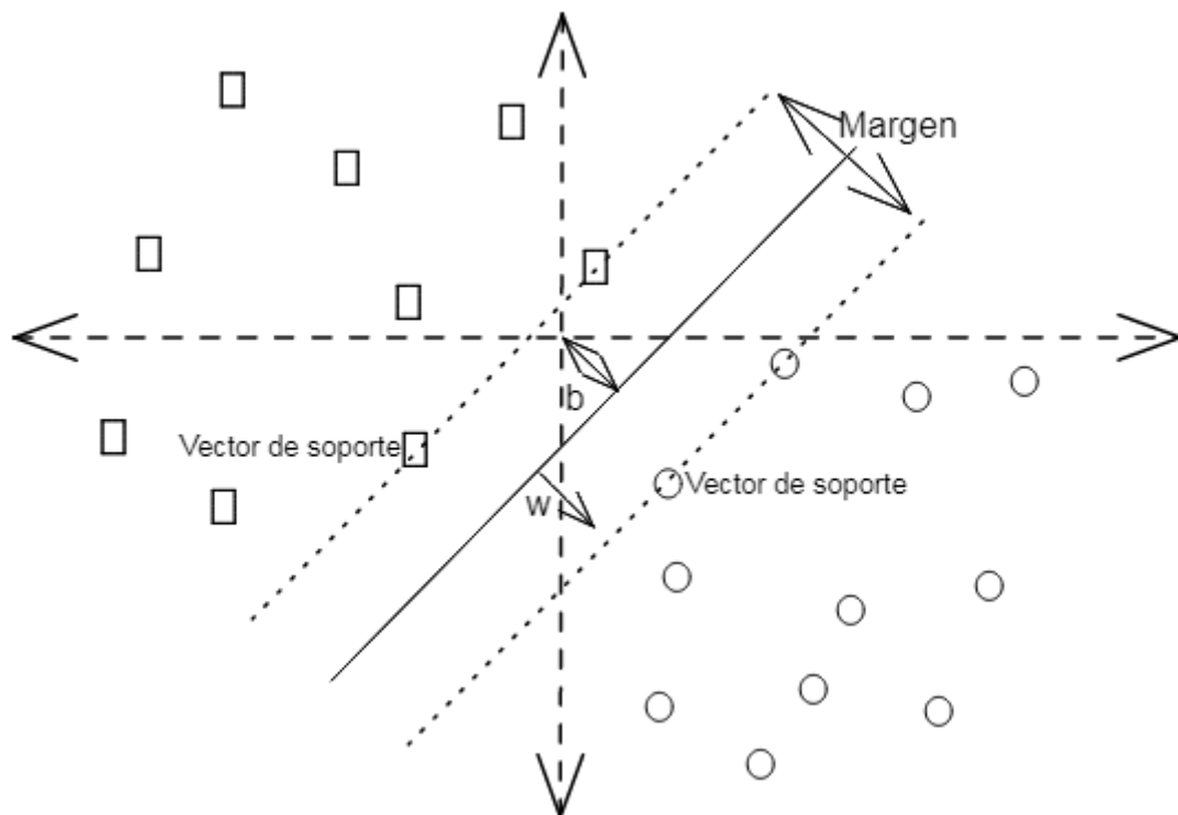
Ilustración 1. Ejemplo de clasificación en dos grupos mediante Linear SVM
