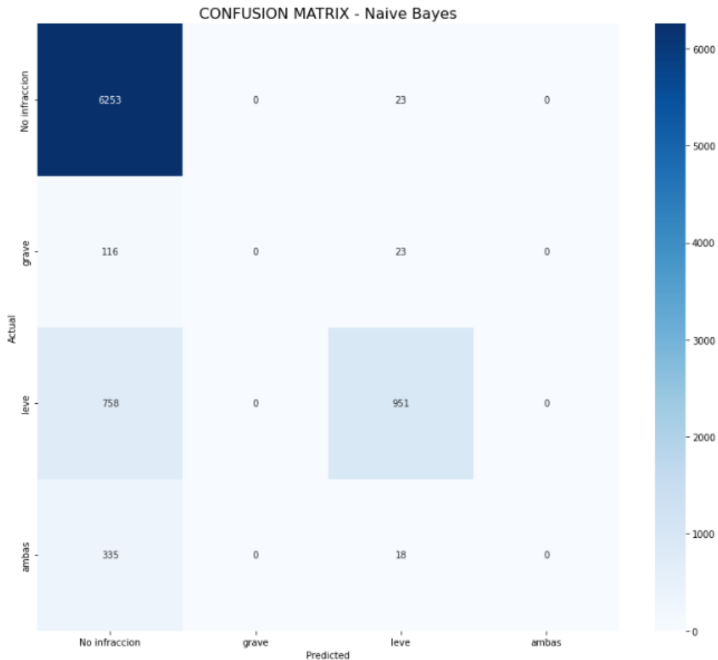
Ilustración 12. Matriz de Confusión para el modelo Naïve Bayes
