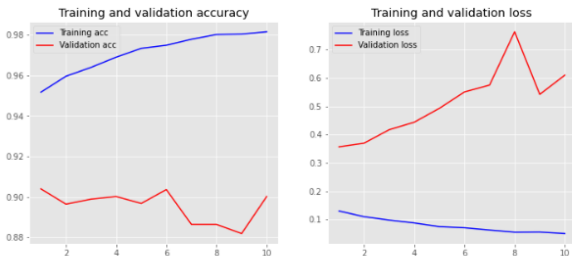
Ilustración 17. Precisión y función de pérdida del modelo para 10 epochs
