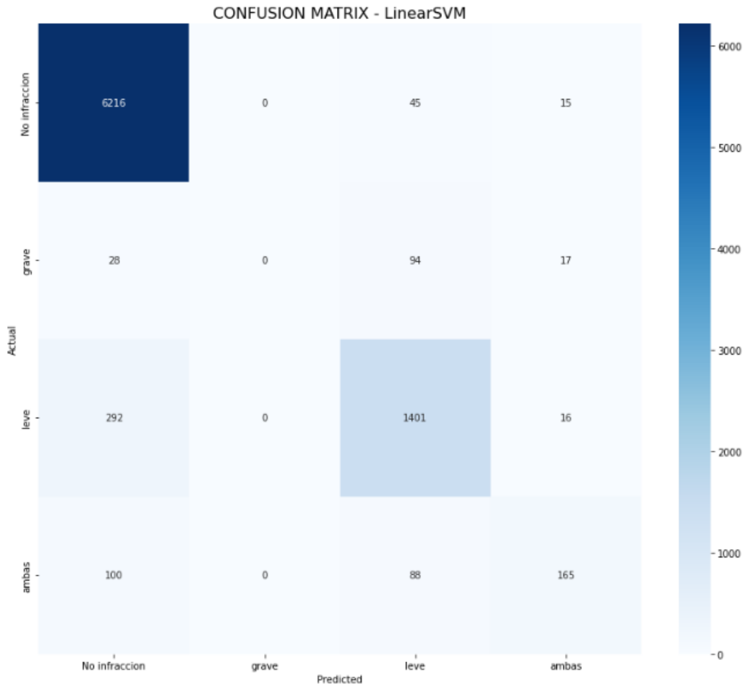
Ilustración 13. Matriz de Confusión para el modelo Linear Support Vector Machine
