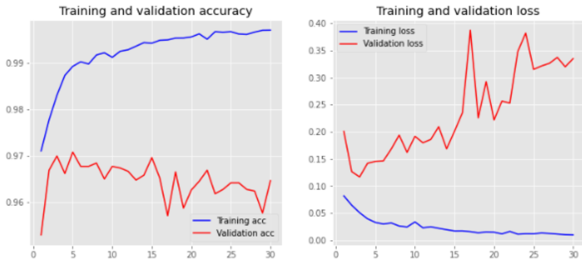
Ilustración 16. Precisión y función de pérdida del modelo para 30 epochs
