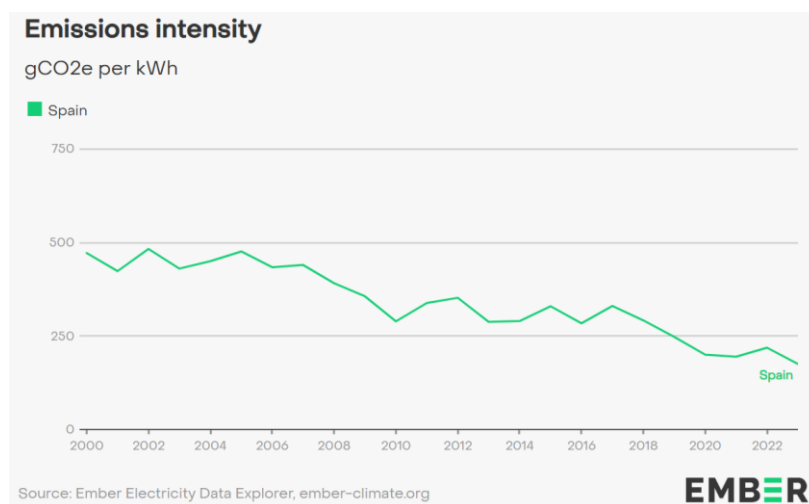
Figura 11: Emisiones gramos CO 2 por kWh [EMBER]
