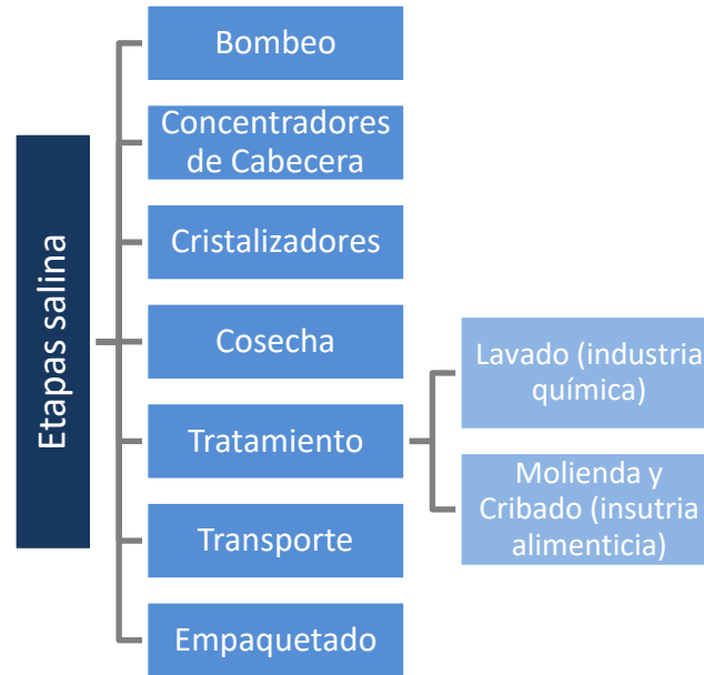
Figura 10: Esquema etapas salina [Elaboración propia]
