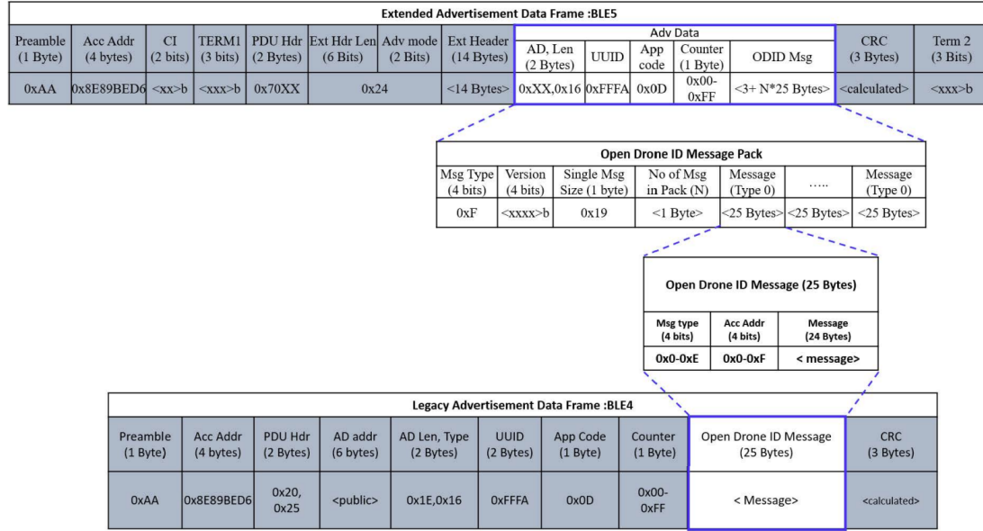
Figura 2.2: Diagrama de la trama del Open Drone ID transmitidos en BLE [12]
