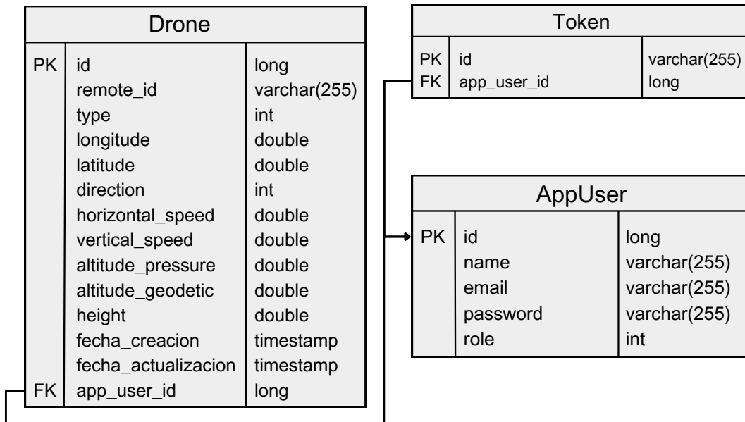
Figura 5.2: Diagrama de base de datos
