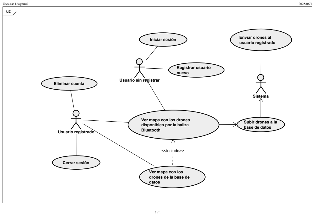
Figura 5.6: Diagrama de casos de uso
