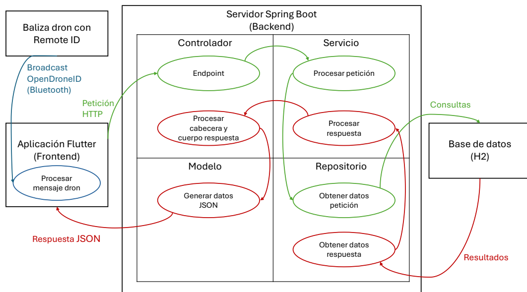
Figura 5.5: Diagrama de caja negra del backend .
