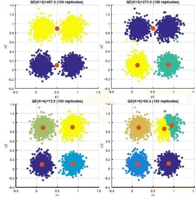
Figura 2.5: K-Means con distinto número de K [17]
