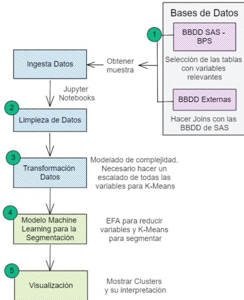
Figura 3.1: Esquema Resumen Arquitectura del Trabajo
