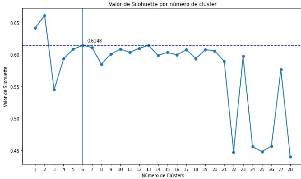
Figura 4.4: Silhouette Analysis: Elección de número de clusters
