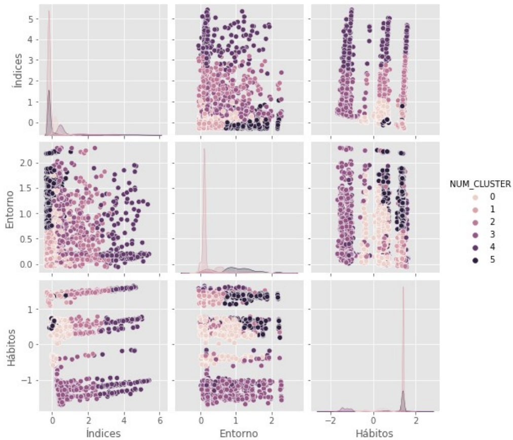
Figura 4.5: Segmentación de los clusters en 2-D
