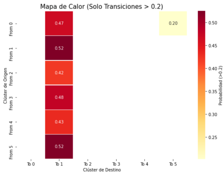
Figura 4.12: Mapa de calor filtrado de las transiciones entre clusters
