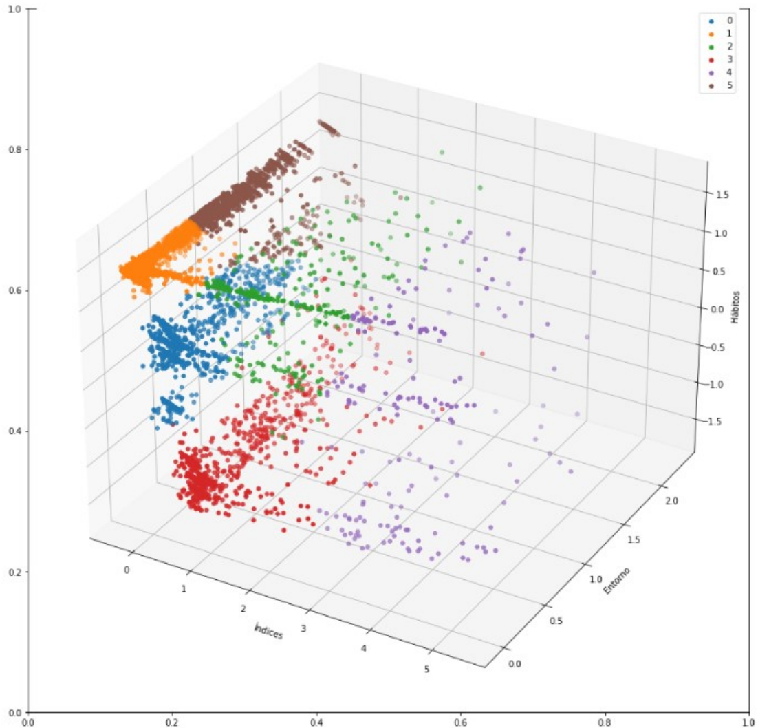
Figura 4.6: Segmentación de los clusters en 3-D
