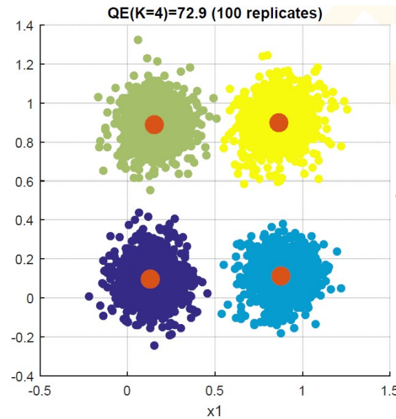
Figura 2.7: K-Means terminado con K=4 para los datos de entrada [17]
