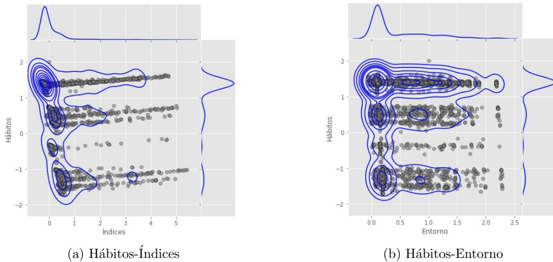
Figura 4.3: Gráficos de Factores tras el Factor Analysis (EFA)
