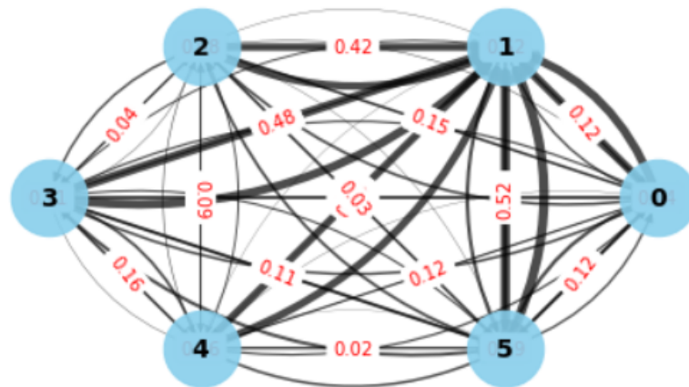
Figura 4.9: Probabilidad de transición entre clusters por Cadenas de Markov
