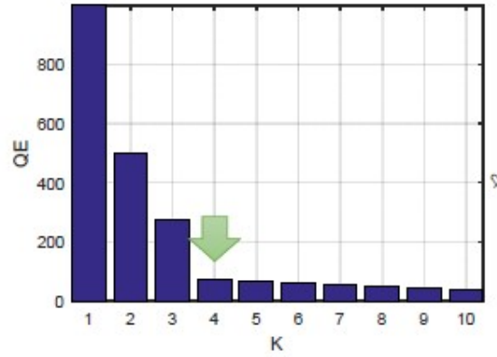
Figura 2.6: Método del codo y QE para la elección de K [17]
