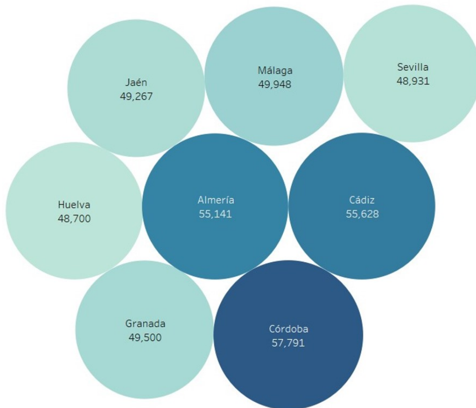
Figura 3.9: Análisis Exploratorio - Edad Media por Provincia
