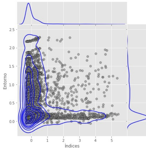
Figura 4.2: Gráfico del Factor Entorno contra el Factor Índices
