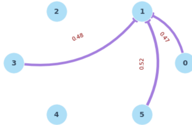
Figura 4.11: Los tres movimientos más probables por Cadenas de Markov
