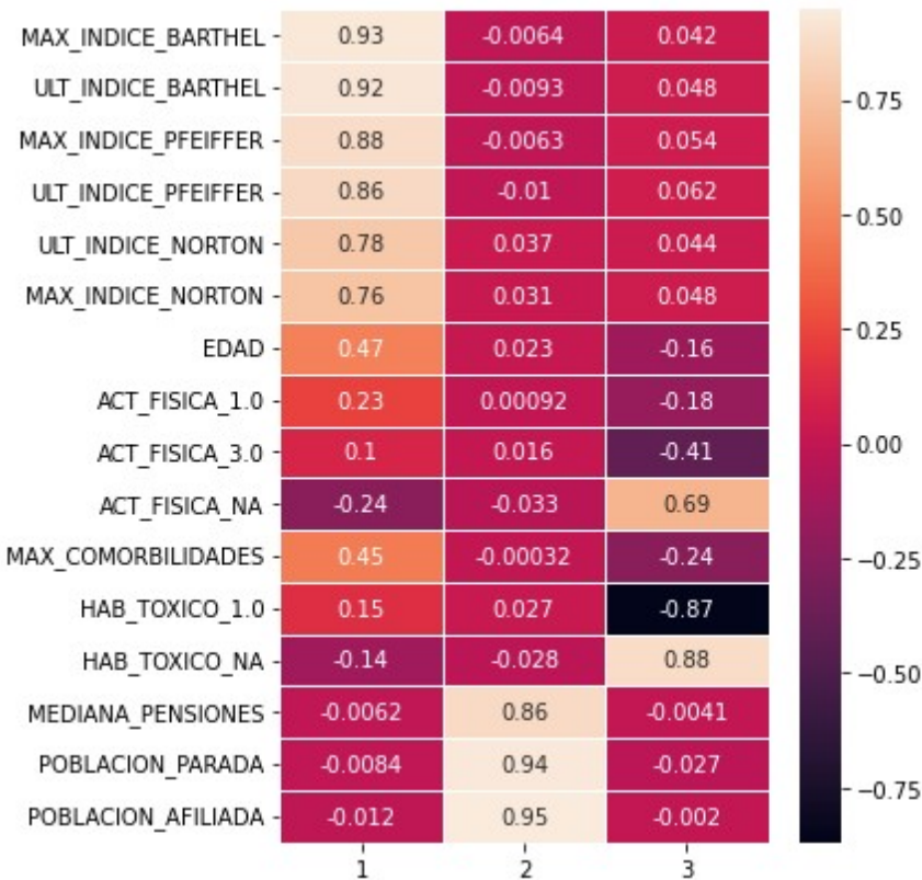
Figura 4.1: Mapa de calor de correlaciones entre variables y los factores
