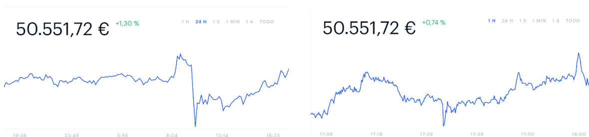
Figura 8. Variaciones del precio de BTC en 1 día y 1 hora
